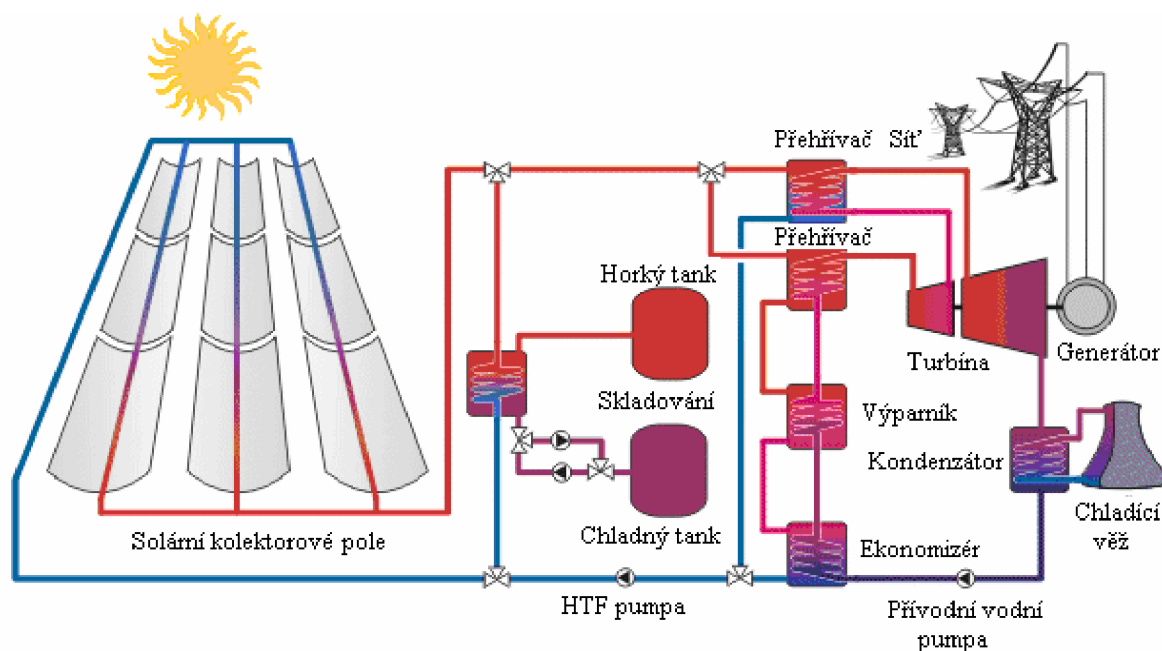
Obrázek 12: Princip fungování žlabové STE s teplotním zásobníkem. [36]
