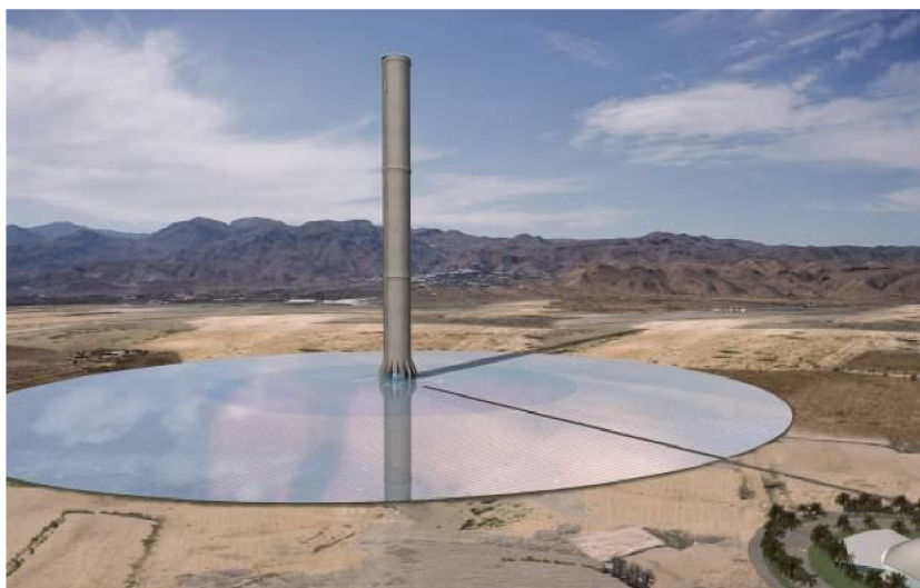
Obrázek 15: Ukázka solární komínové elektrárny. [36]
