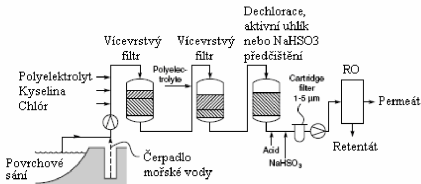
Obrázek 24: Proces předúpravy vody a RO. [51]
