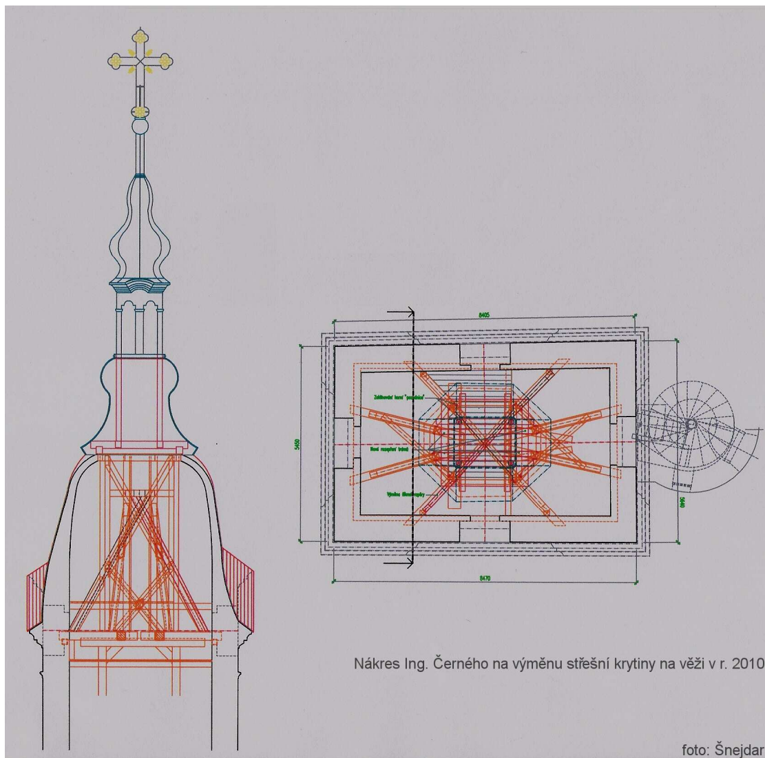
Nákres Ing. Černého na výměnu střešní krytiny na věži v r. 2010
