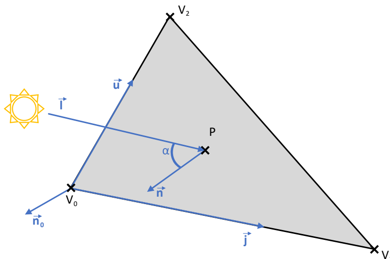
Obr. 4.5: Výpočet u konštantného tieňovania, prevzaté z [1].
