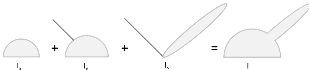
Obr. 4.3: Odrazené svetlo vo Phongovom modeli osvetlenia. Ambientná, difúzna a zrkadlová zložka sa sčítajú do konečného odrazu, prevzaté z [1].
