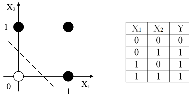
Obrázek 2.4: Funkce OR, ukázka lineárně separovatelných dat
