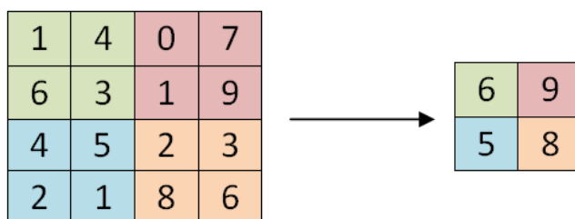
Obrázek 2.8: Schéma max-poolingu
