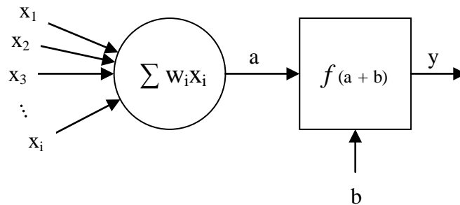
Obrázek 2.2: Schéma perceptronu
