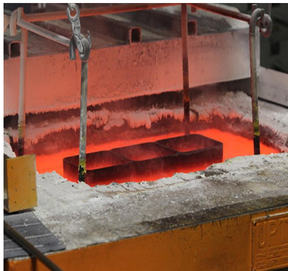
Obr. 33 Solná lázeň [50]
