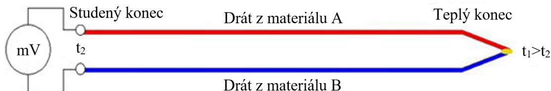
Obr. 6 Princip termočlánků [12]
