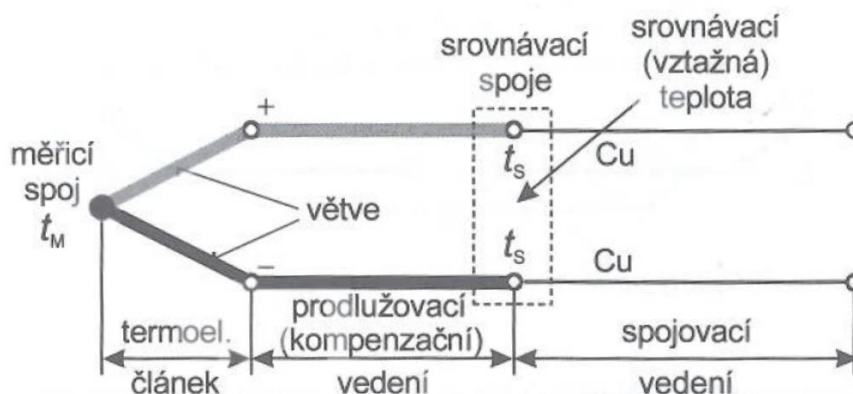
Obr. 16 Schéma zapojení [11]
