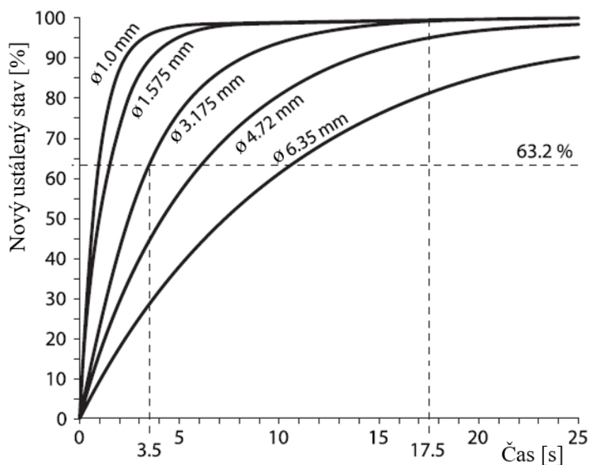
Obr. 12 Časové konstanty [31]
