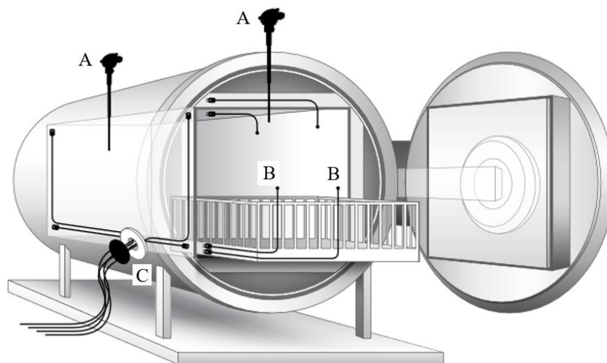
Obr. 30 Vytvrzovací pec [18]
