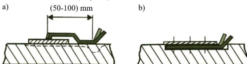
Obr. 24 Měření povrchové teploty [11]
