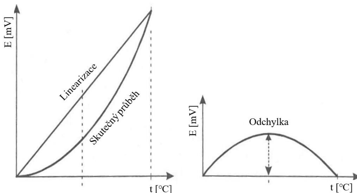
Obr. 7 Nelinearita [11]
