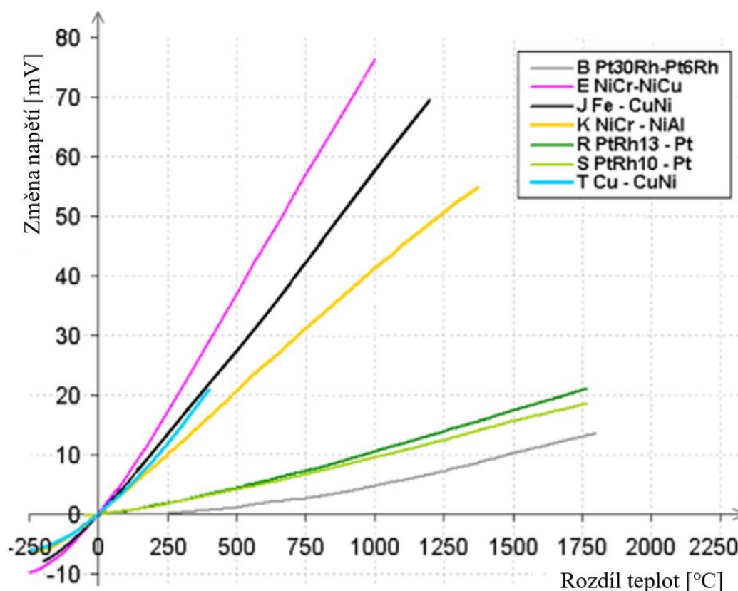
Obr. 8 Charakteristiky [19]
