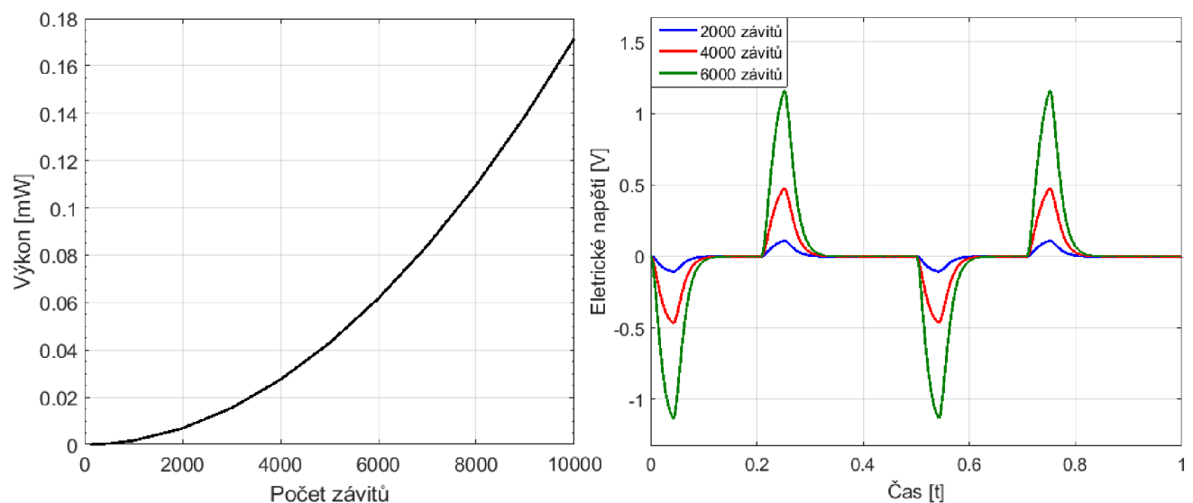
Obrázek 51: Závislost středního výkonu na počtu závitů
