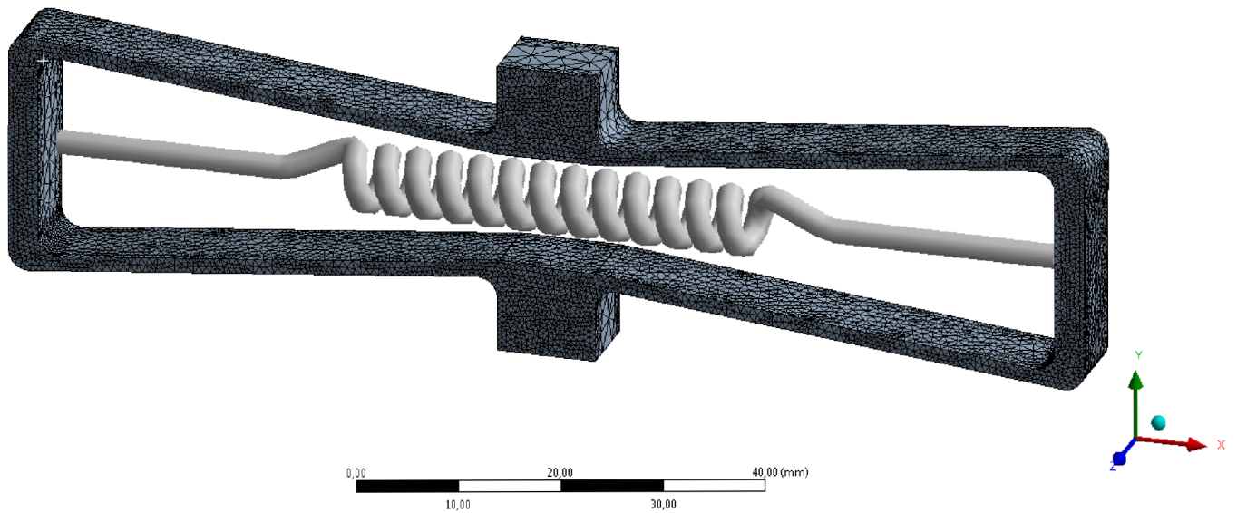
Obrázek 35: MKP síť
