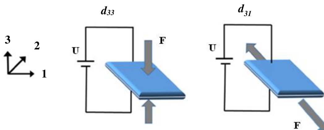
Obrázek 10: Módy piezo-generátorů [33]
