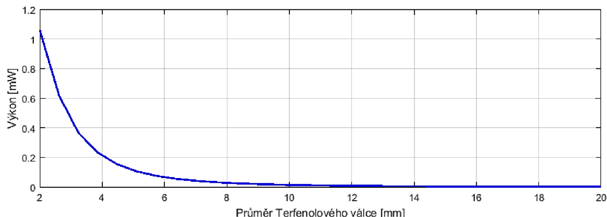
Obrázek 52: Závislost středního výkonu na průměru Terfenolového válce
