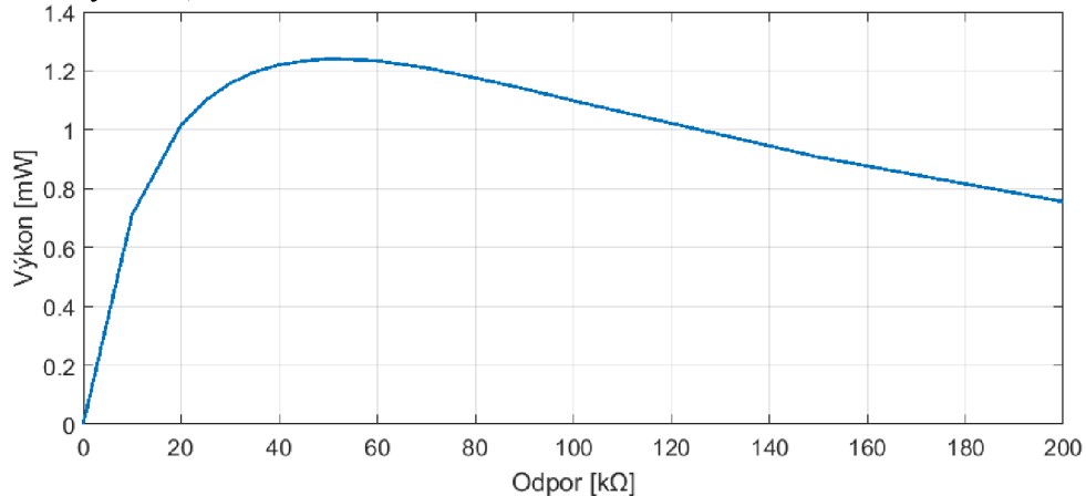
Obrázek 47: Závislost středního výkonu na odporu zátěže
