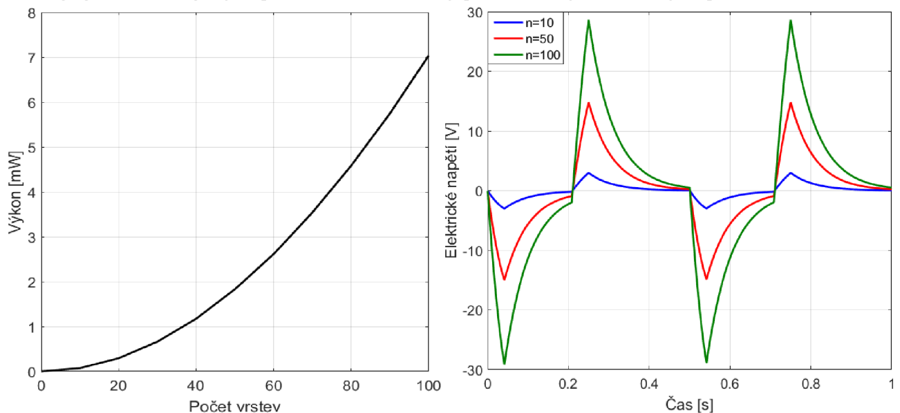
Obrázek 48: Vliv počtu piezoelektrických vrstev na střední výkon a elektrické napětí
