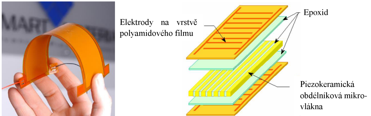
Obrázek 8: Mikro-vláknový kompozit [31]
