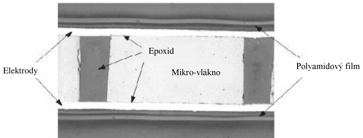
Obrázek 9: Řez kompozitem [32]
