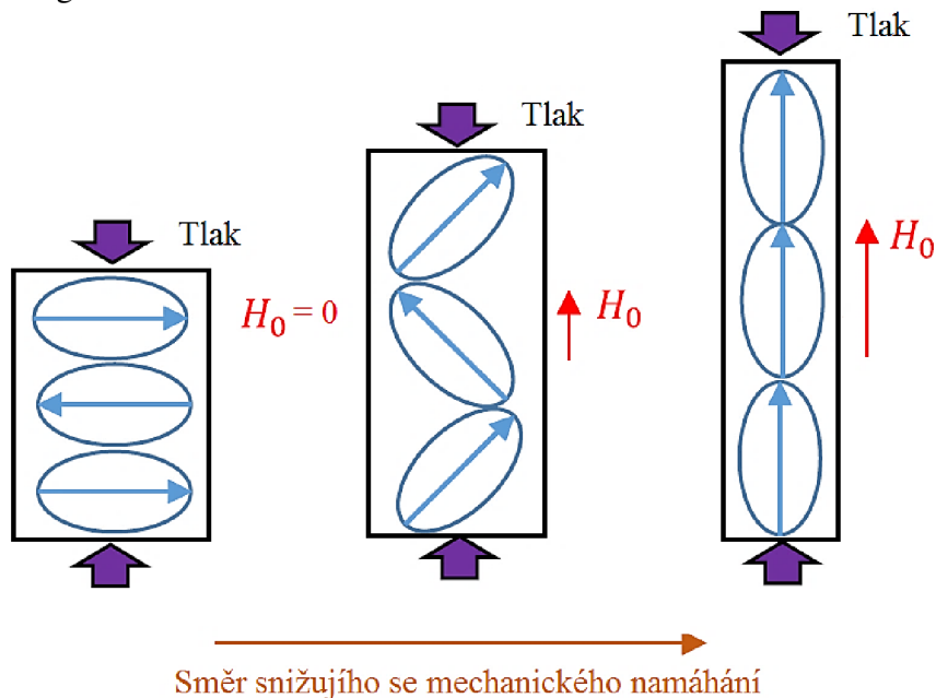
Obrázek 23: Villariho jev [15]
