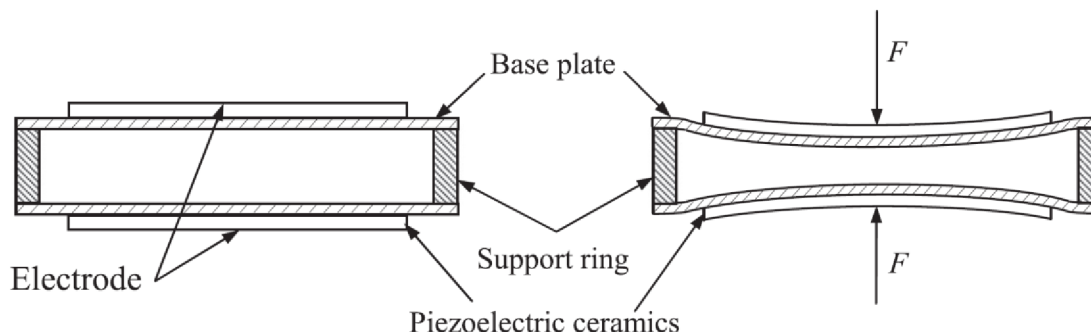
Obrázek 14: Piezoelektrický generátor [18]
