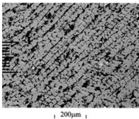
Obrázek 24: Struktura Terfenolu-D [36]
