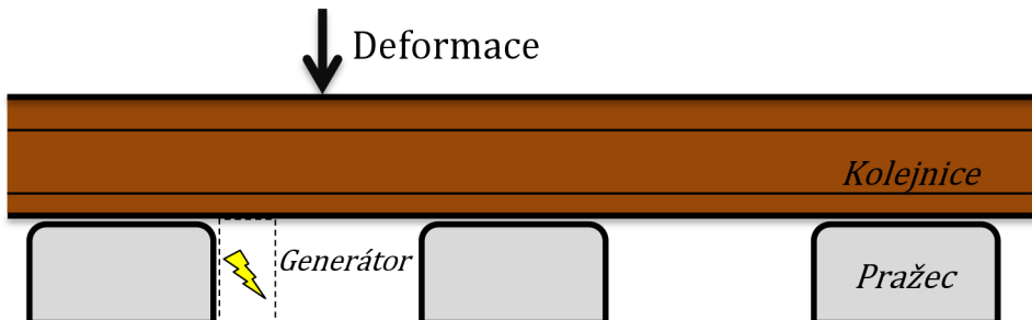
Obrázek 30: Umístění generátoru
