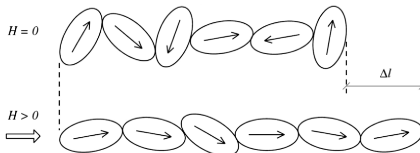
Obrázek 22: Joulův jev [14]
