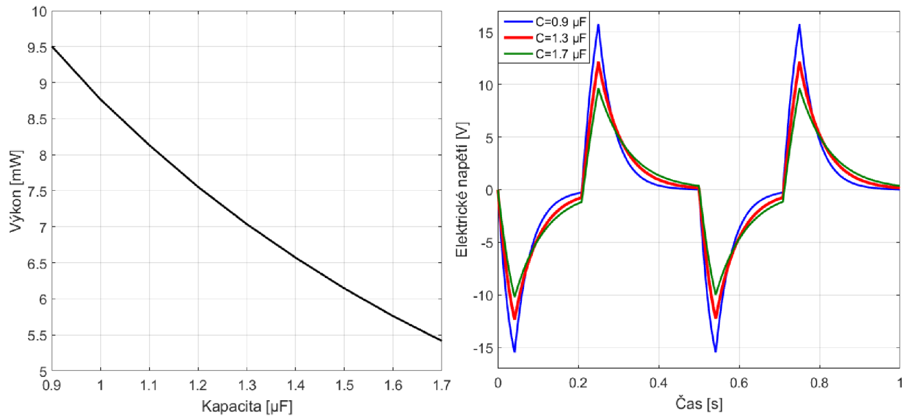
Obrázek 49: Vliv kapacity piezoelektrického stacku na střední výkon a elektrické napětí
