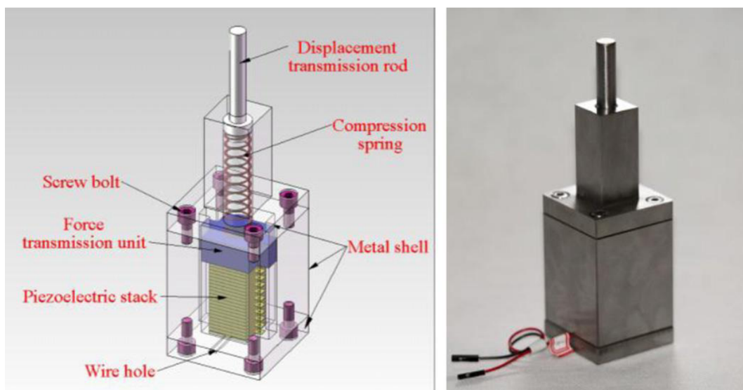
Obrázek 17: Stack-type piezoelektrický generátor [19]
