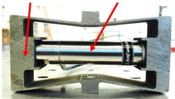
Zesilovací rám Piezoelektrický válec
