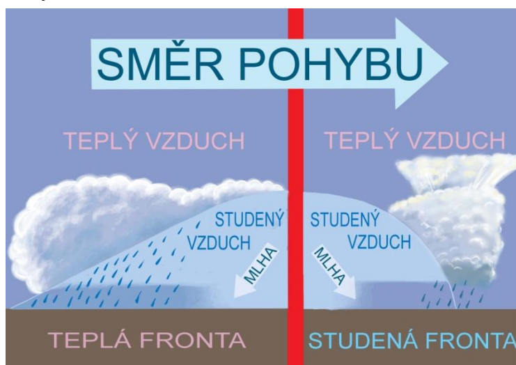
Obr. 2 Frontální mlhy [4]
