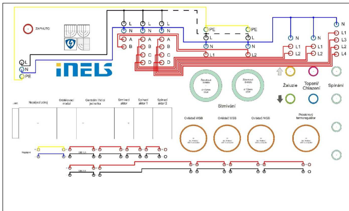
Obr. 5-2: Schéma zapojení panelu
