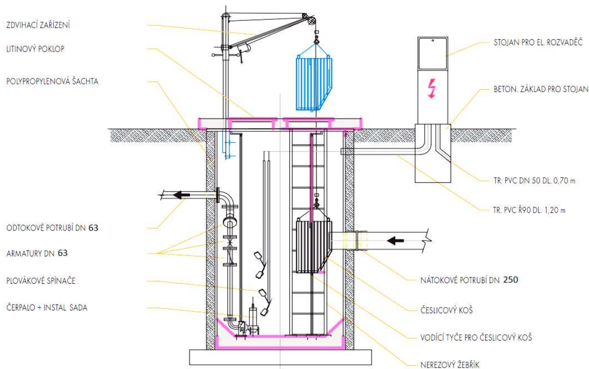
Obr. 4.2 Vystrojení čerpací stanice [30]
