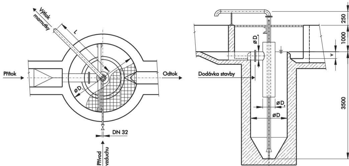
Obr. 4.4 Schéma lapáku písku [32]
