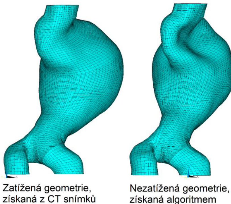
Obrázek 23: Porovnání originální geometrie z CT snímků (vlevo) a nové nezátížené geometrie
