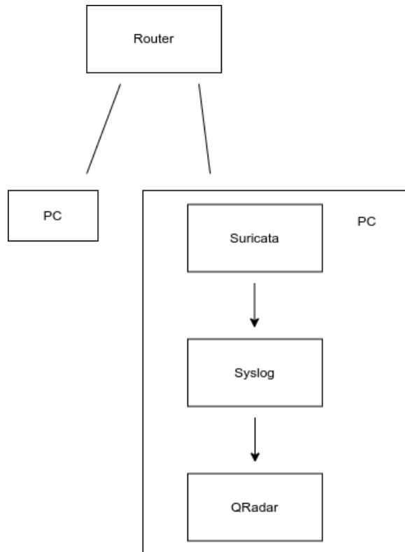
Obr. 6.1: Vizualizácia jednotlivých prvkov v sieti
