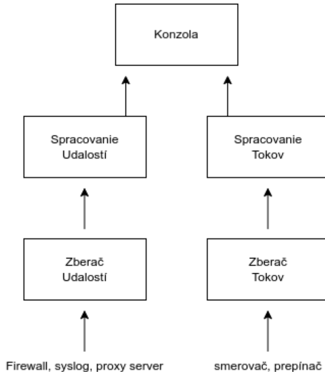
Obr. 3.1: Základná architektúra programu IBM QRadar
