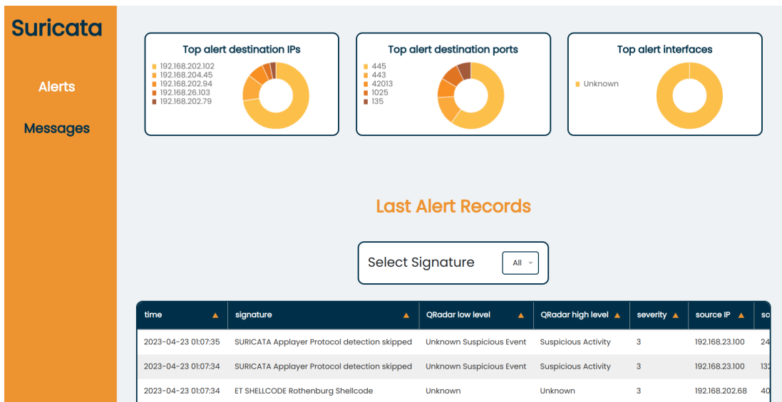
Obr. C.4: Grafy a začiatok tabuľky
