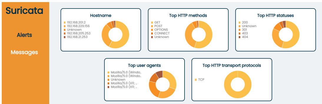
Obr. C.9: Grafy zobrazujúce údaje o type udalosti HTTP
