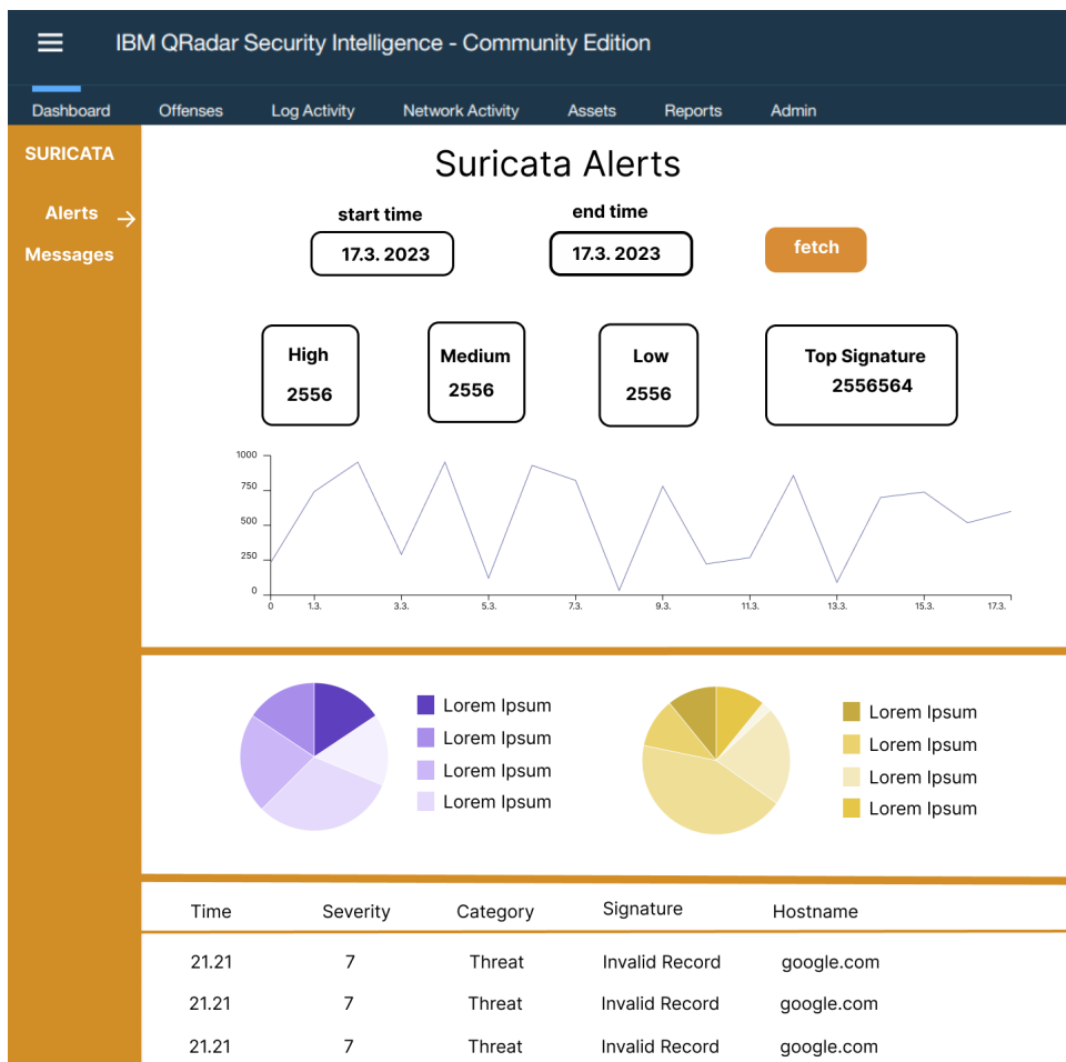
Obr. 5.3: Návrh karty pre hrozby vo figme
