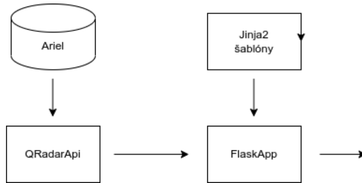
Obr. 5.2: Štruktúra navrhovaného add-on
