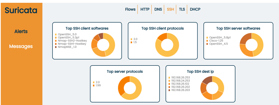
Obr. C.11: Grafy zobrazujúce údaje o type udalosti SSH
