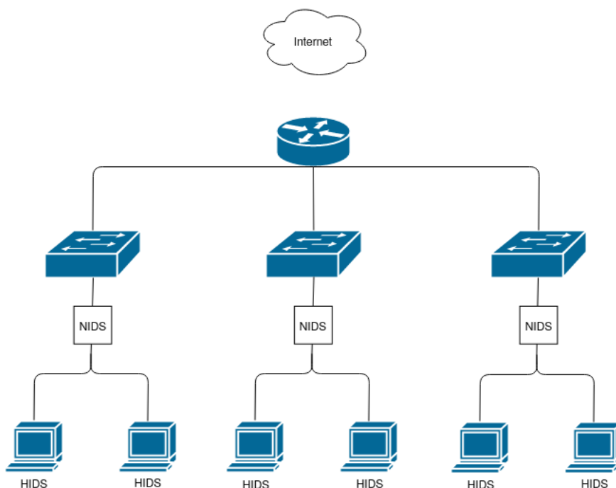
Obr. 2.1: Rozloženie HIDS a NIDS v sieti [7]
