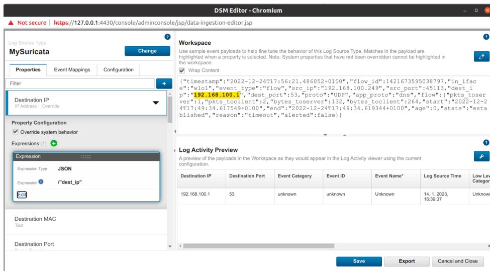
Obr. 6.2: Modálové okno pre konfiguráciu DSM
