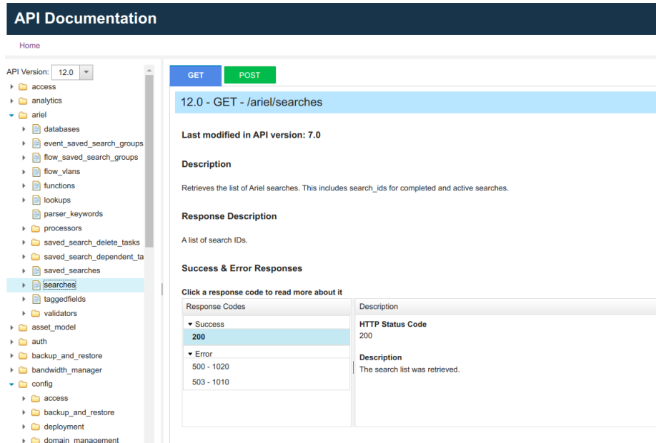
Obr. 3.2: Screenshot z dokumentácie QRadar REST API
