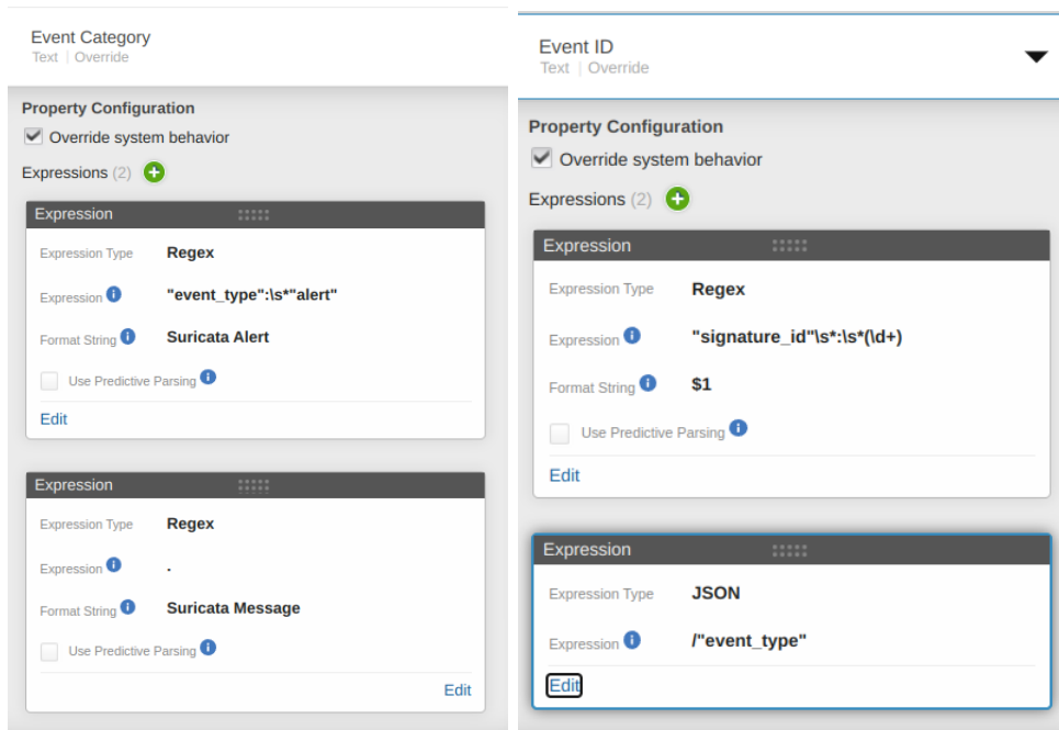
Obr. 4.1: Snímka regulárnych výrazov kategórie a identifikátora udalostí
