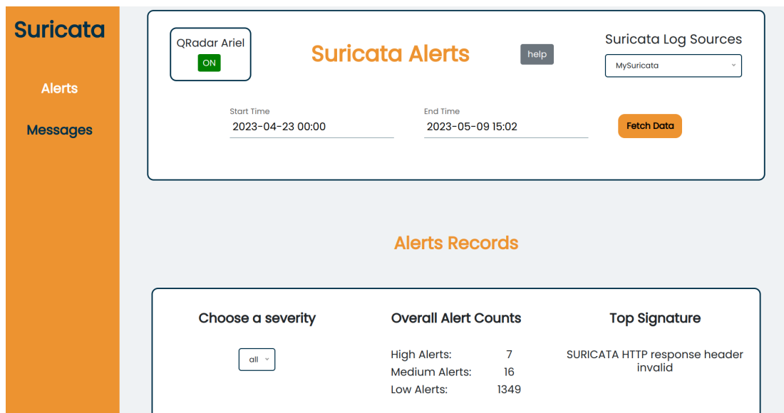
Obr. C.1: Vzhľad vrchného panelu karty hrozby
