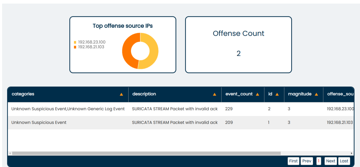
Obr. 7.9: Zobrazenie hrozieb v systéme
