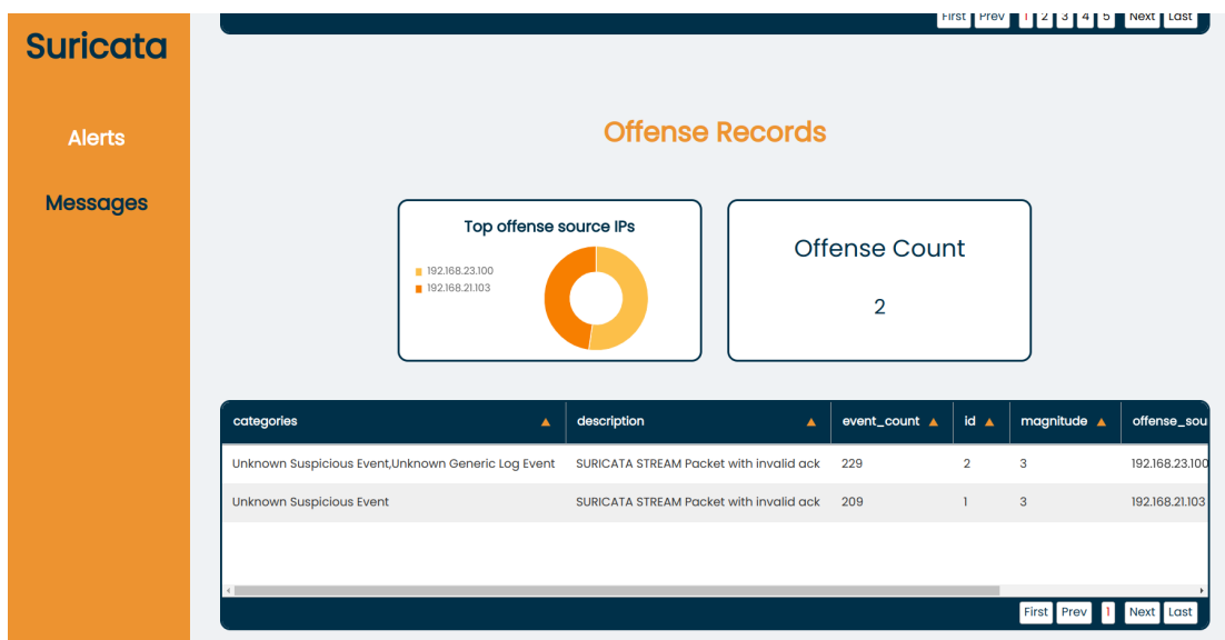
Obr. C.6: Časť karty hrozby zobrazujúca informácie o priestupkoch
