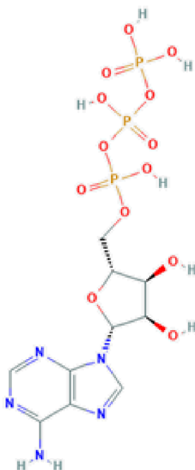
Obrázek 4. Struktura adenosintrifosfátu [30]
