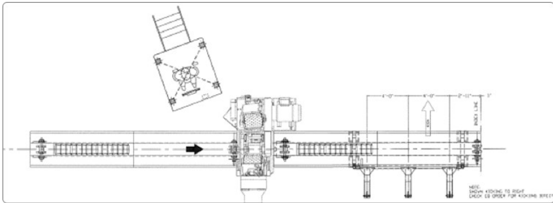
Obrázek 4 Schéma odkorňovače
