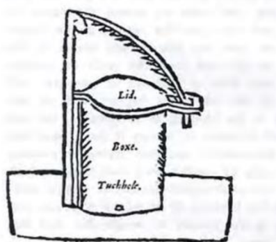
Obrázek č. 5: Bournivův přístroj určený k testování účinnosti černého prachu (Muller 1973)
