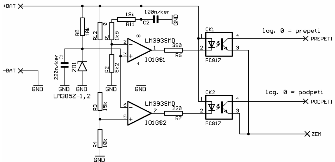
Obr. 5.4.2: Schéma zapojení obvodu komparátorů
