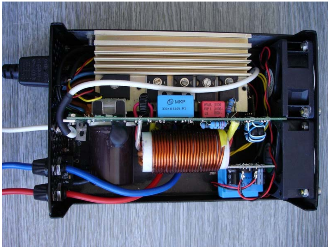
Obr.8.1: Sestavená nabíječka
