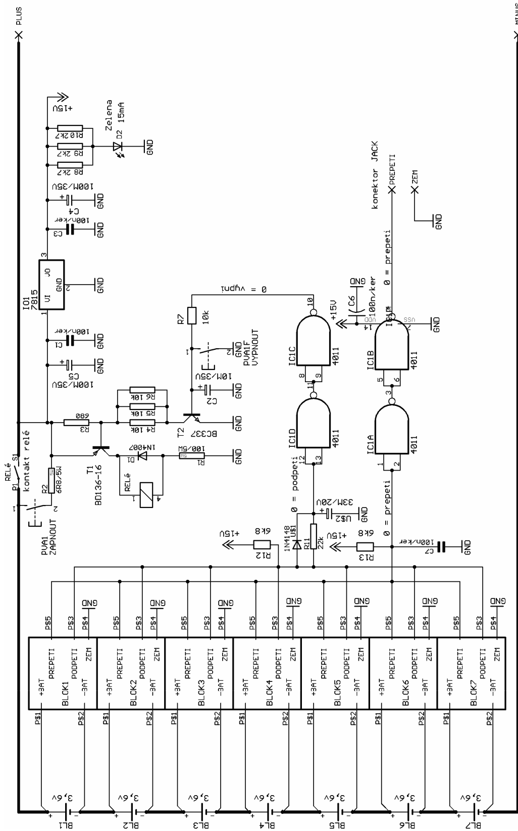
Obr. 5.4.1: Schéma zapojení ochranných obvodů
