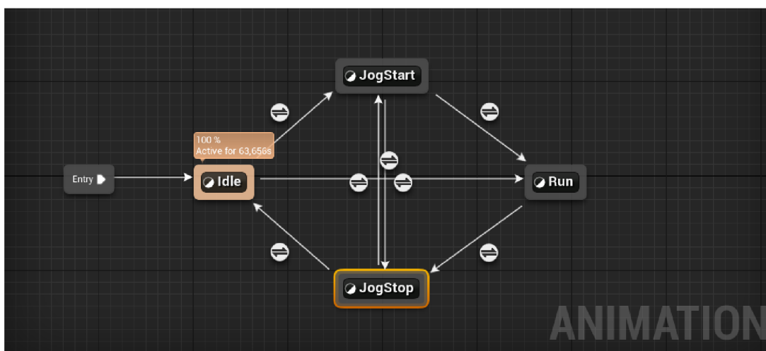
Obrázek 25: Stavový diagram, který řídí animace nohou.
