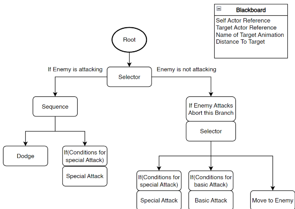
Obrázek 36: Diagram rozhodování pokročilé umělé inteligence.
