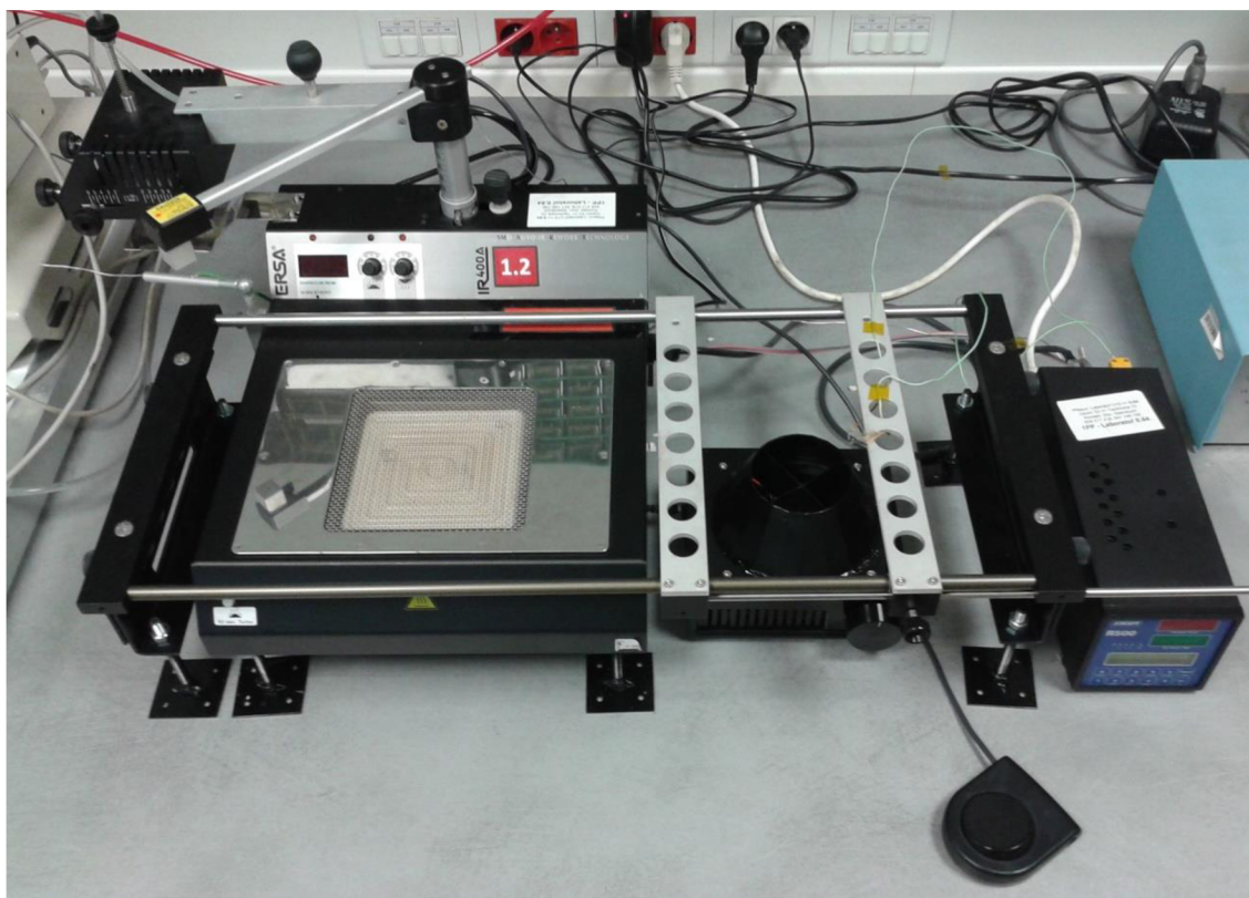
Obrázek 6.1: Opravárenská stanice Erska IR-400.
