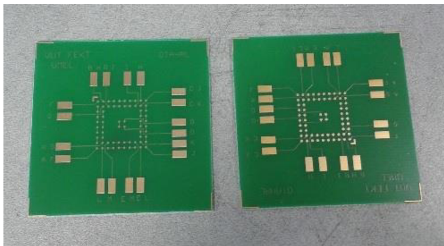
Obrázek 3.1: Substrát FR4.
