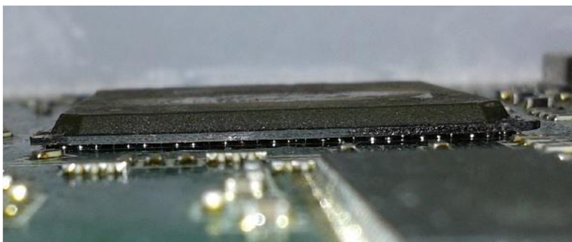
Obrázek 9.3: Optická kontrola zapájení testovacího BGA.
