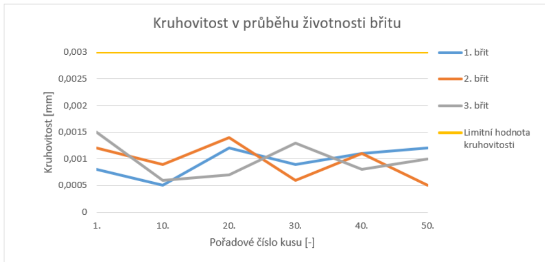
Obr. 47 Grafická interpretace naměřených hodnot kruhovitosti v průběhu životnosti břítu.
