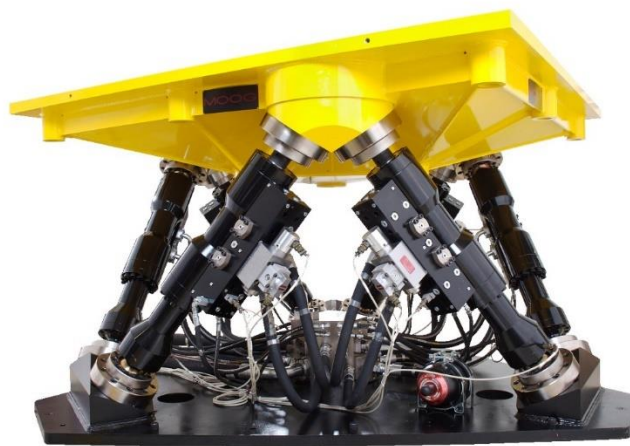
Obr. 1 Simulační hydraulická stolice [2].
