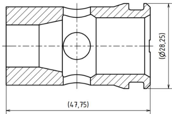
Obr. 6 Vlevo řez vyráběného kartušového ventilu a vpravo jeho model, po obrobění první polohy.
