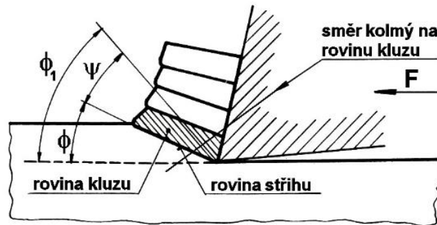
Obr. 17 Schéma rovin v procesu tvorby třísky [16].
