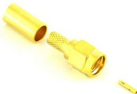
Obr. 2.15: Rozmontovaný konektor R-SMA
