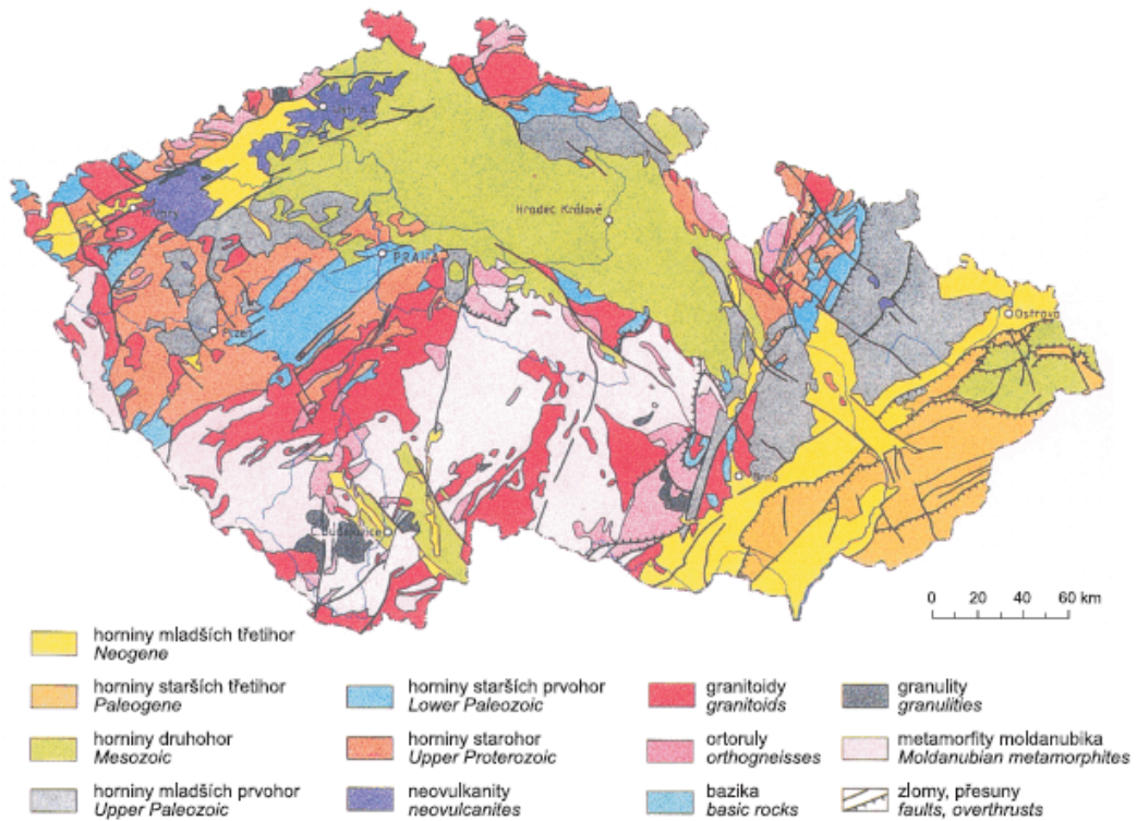
Obr. č. 4 Geologická mapa ČR (Chlupáč et al., 2002)
