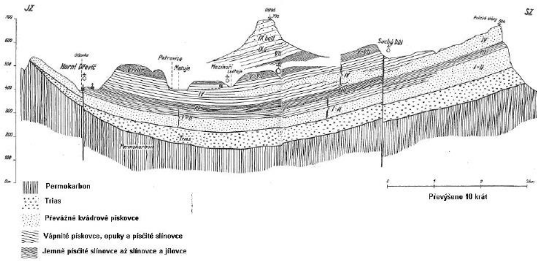
Obr. č. 3 Průřez Polickou pánví (Kunský, 1986)
