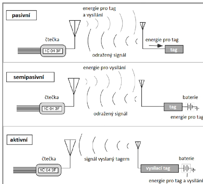
Obr. 4: Rozdělení tagů na aktivní, semipasivní, pasivní – převzato z [2]
