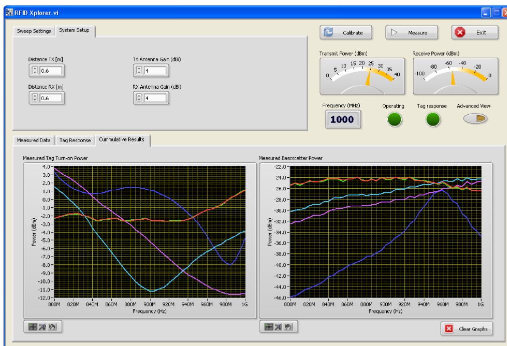
Obr. 18: Softwarové vybavení měřicího systému RFID Xplorer®
