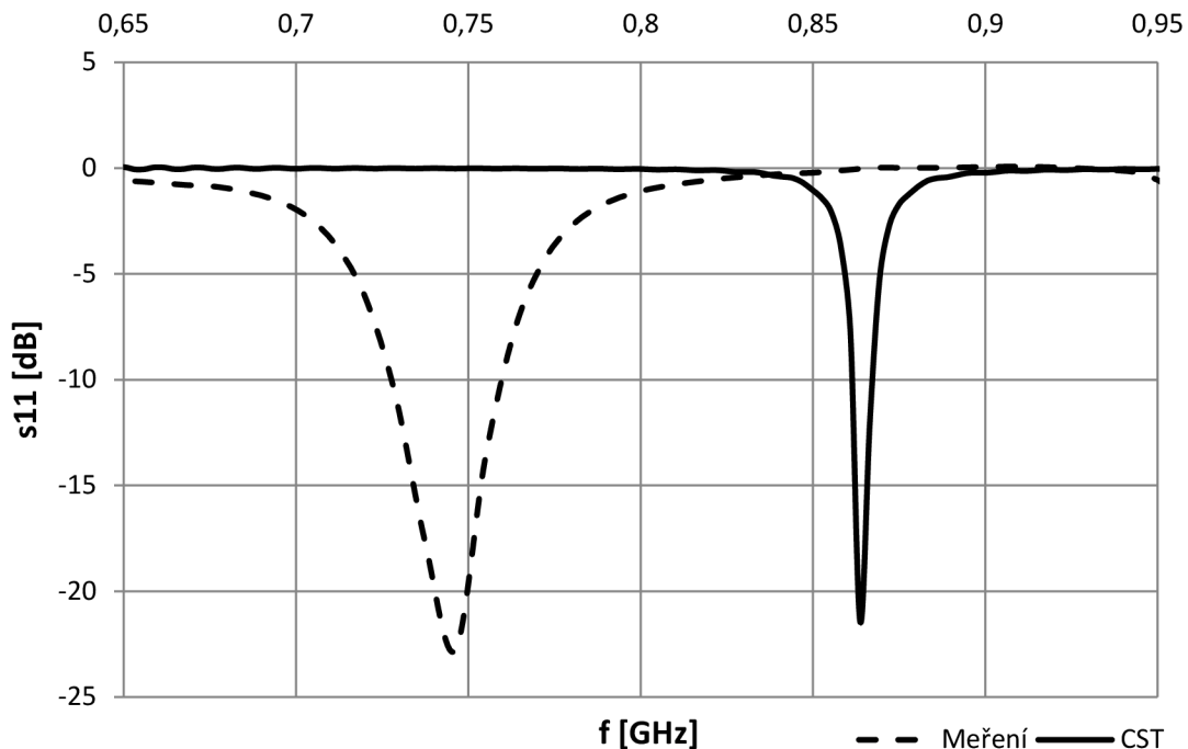
Obr. 35: Závislost činitele odrazu na frekvenci
