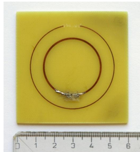
Dvoukruhová anténa
