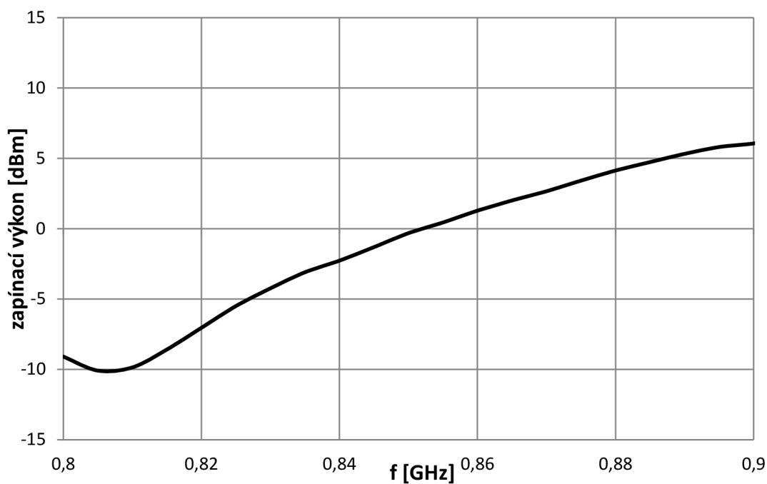
Obr. 37: Výkon nutný pro zapnutí tagu
