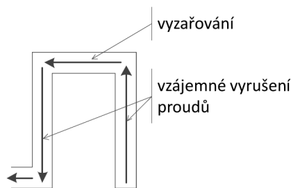
Obr. 16: Proud v sousedních ramenech meandrové struktury
