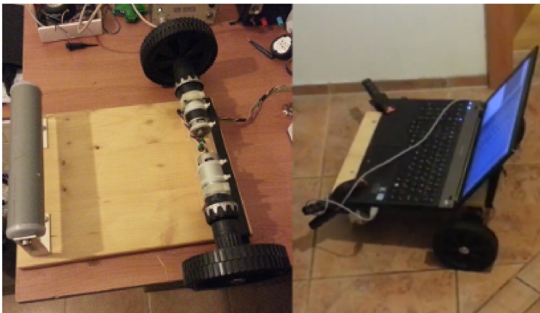
Obrázek 5.3: Fotky druhého prototypu robota.
