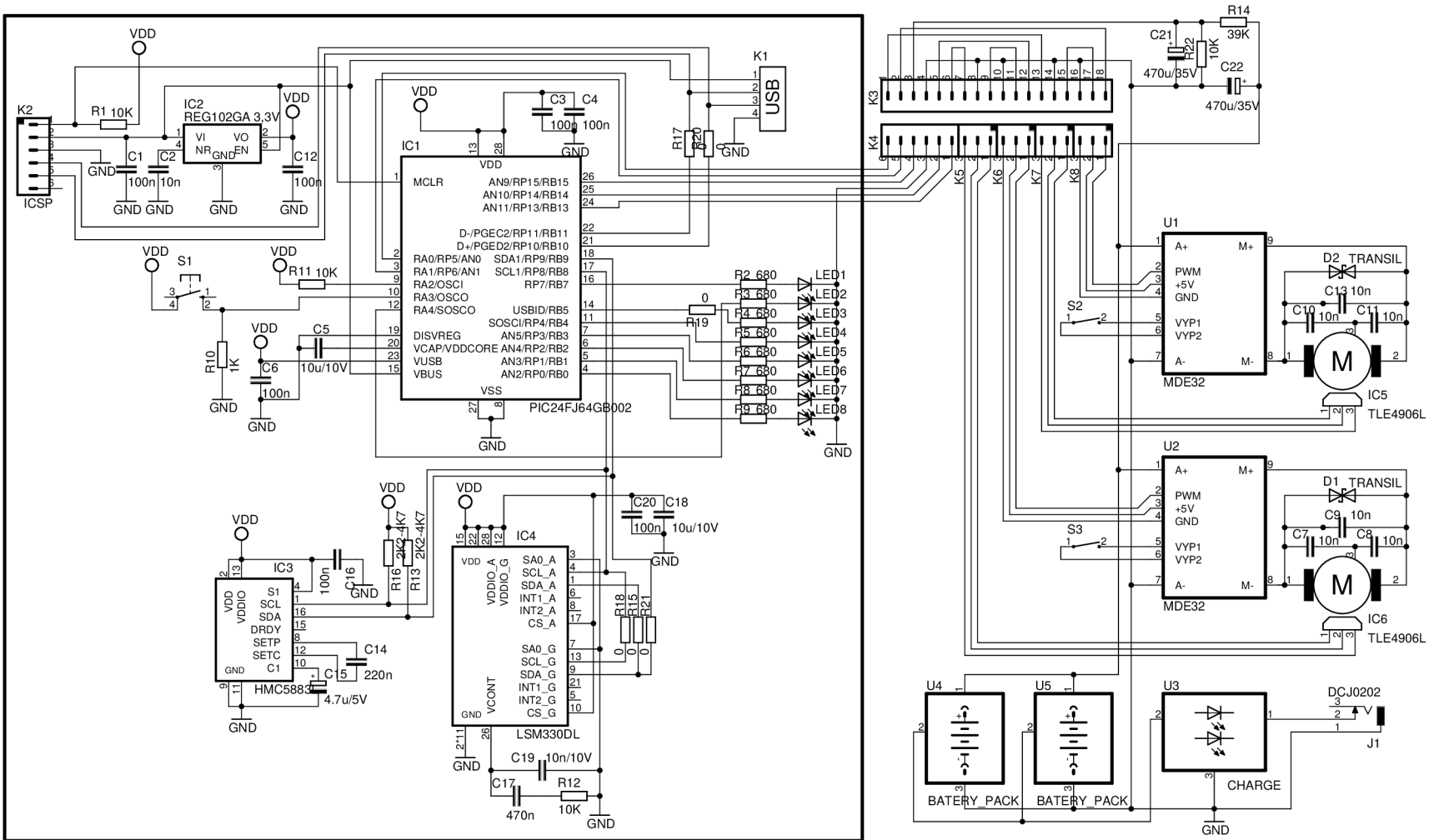
Obrázek A.2: Schéma zapojení druhého prototypu řídicí a senzorové jednotky. 65
