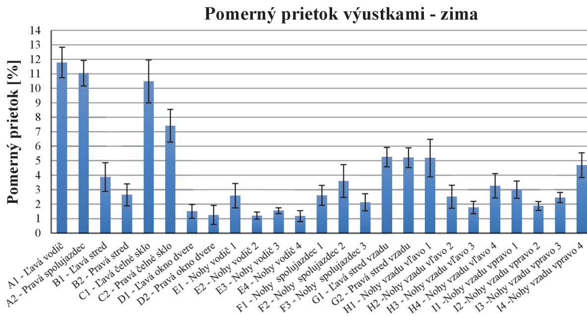
graf 7.5 Pomerný objemový prietok jednotlivými výstmkami so zobrazením chybových úsečiek rozšírenej neistoty - zima
