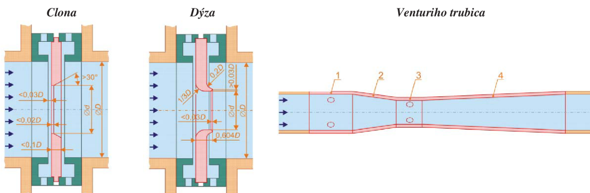
obrázok 4.3 Škrtiace prvky [4]
