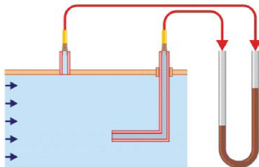
obrázok 4.7 Pitotova trubica [4]
