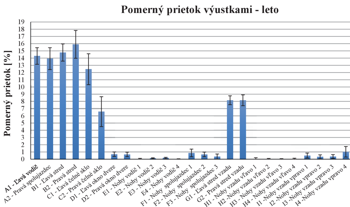
graf 7.1 Pomerný objemový prietok jednotlivými výstmkami so zobrazením chybových úsečiek rozšírenej neistoty - leto
