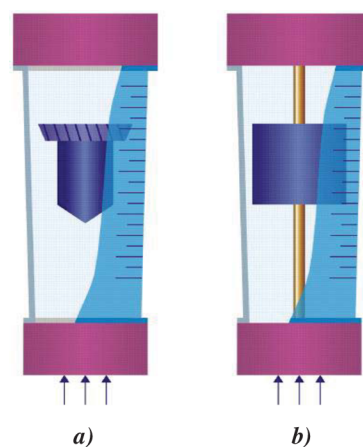
obrázok 4.4 Plavákový prietokomer [4] a) so stabilným plavákom b) s nestabilným plavákom
