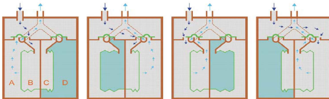
obrázok 4.2 Suchý plynomer [4]
