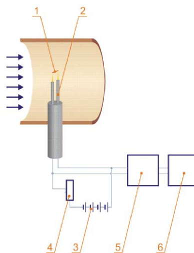
obrázok 4.9 Žeraviaci anemometer s kovovým vláknom, metóda CCA [4]
