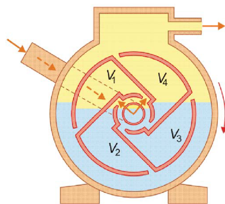
obrázok 4.1 Mokrý plynomer [4]
