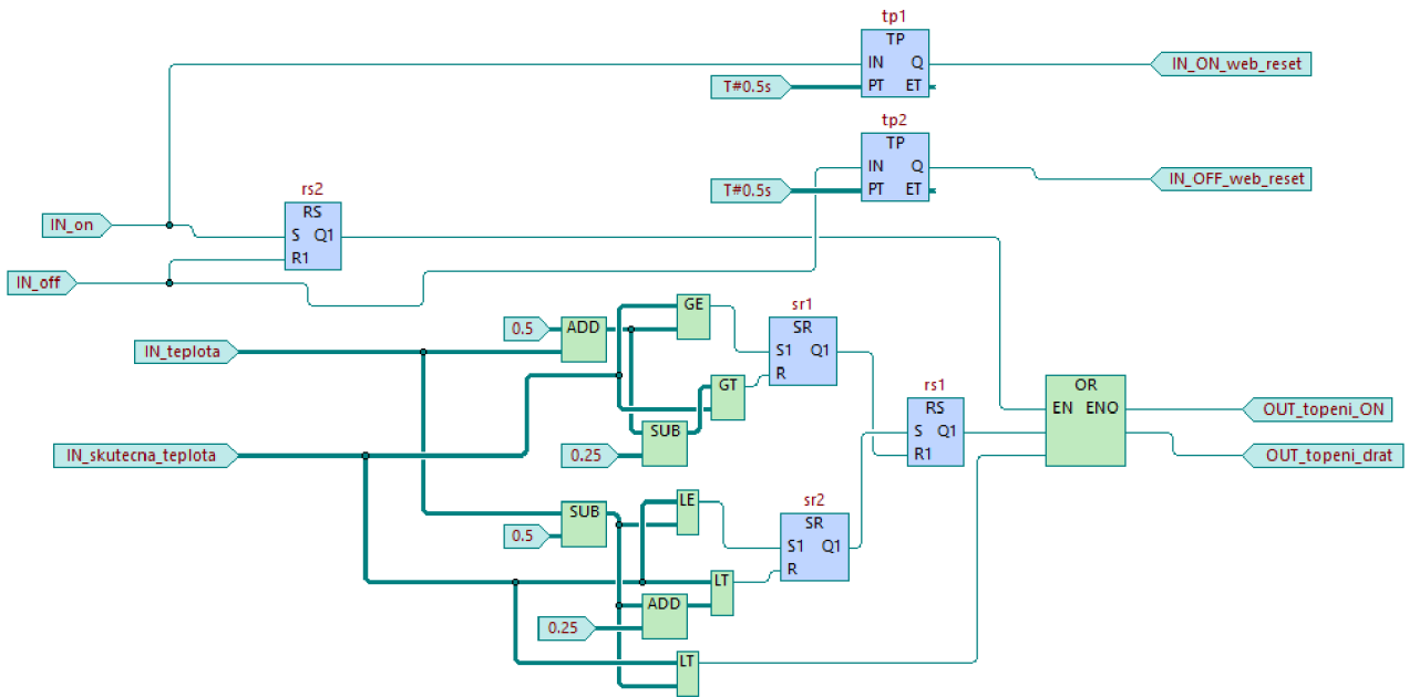
Obrázek 6-16 - Vnitřní zapojení termostatu topení
