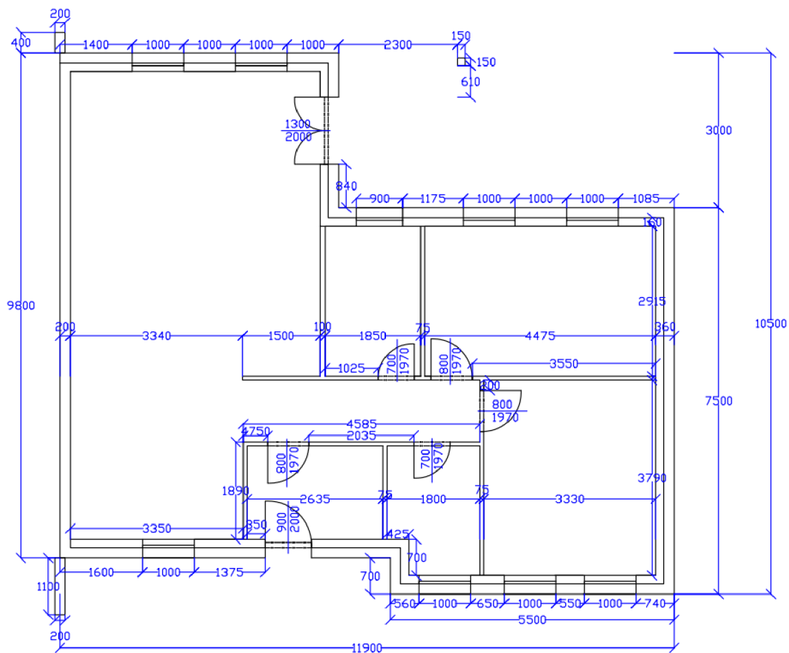
Obrázek 4-1- Půdorys domu
