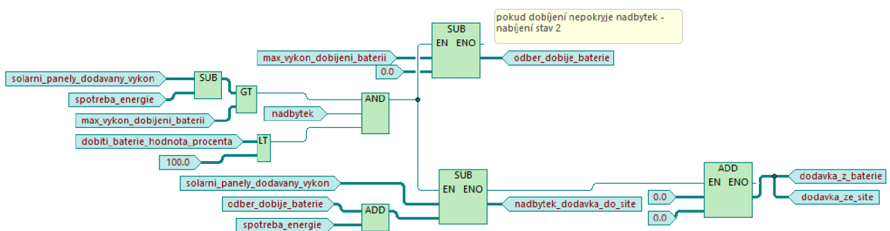
Obrázek 6-17 - Ukázka z energetického managementu, stav nadbytku 2. stupně
