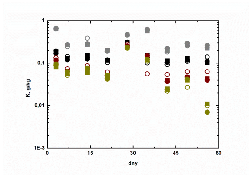
Obrázek 5.5 Závislost množství draslíku na délce trvání inkubačního pokusu (○–vzorek bez papercharu, ●–vzorek s papercharem tvořeným suspenzí biocharu, vermitea a roztokem hnojiv, ■–vzorek s papercharem tvořeným suspenzí biocharu, vermitea a hnojiv, ●–zemědělská půda, ●–lesní půda, ●–sterilní půda, ●–písek)
