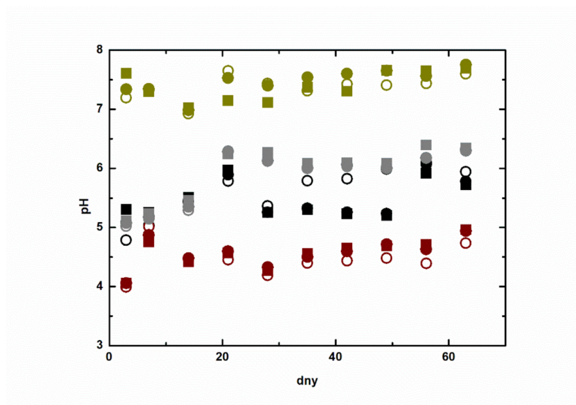
Obrázek 5.1 Závislost pH na délce trvání inkubačního pokusu (○—vzorek bez papercharu, ●—vzorek s papercharem tvořený suspenzí biocharu, vermitea a roztokem hnojiv, ■—vzorek s papercharem tvořeným suspenzí biocharu, vermitea a hnojiv, ●—zemědělská půda, ●—lesní půda, ○—sterilní půda, ●—písek)
