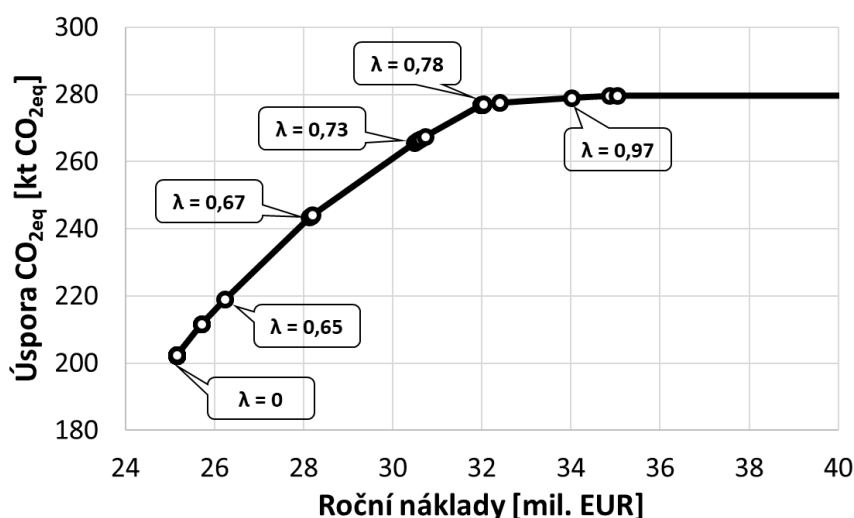
Obr. 4.17: Pareto optimální řešení pro infrastrukturu zpracování plastů.
