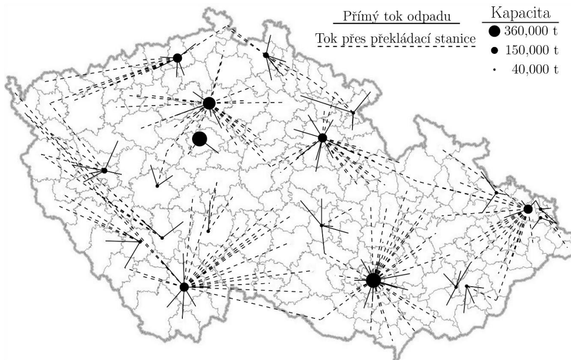
Obr. 4.8: Výsledná mapa toků SKO a rozmístění ZEVO.
