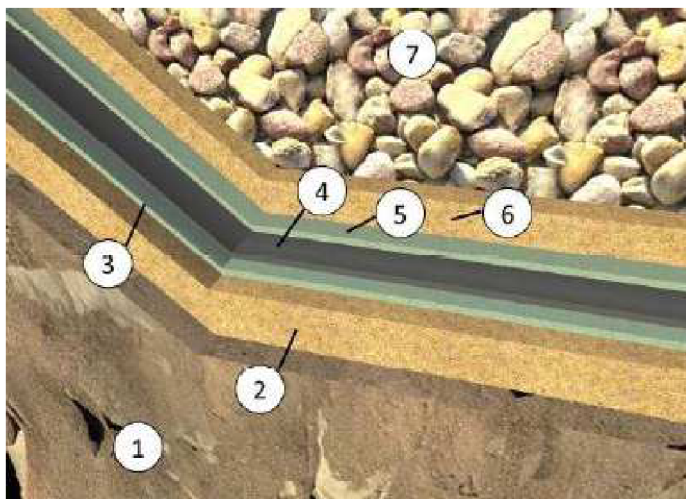
Obr. 9.7 Složení hydroizolační vrstvy: 1 - podloží, 2 - pískový podsyp, 3 - geotextilie, 4 - fólie, 5 - geotextilie, 6 - pískový zásyp, 7 - těleso filtru [15]
