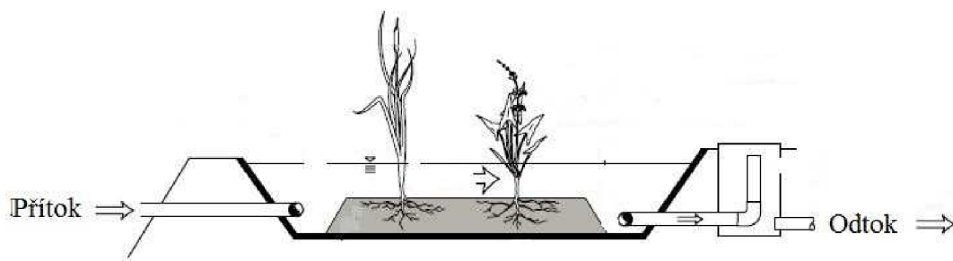
Obr. 3.1 Horizontální kořenová čistírna s površovým průtokem [5]
