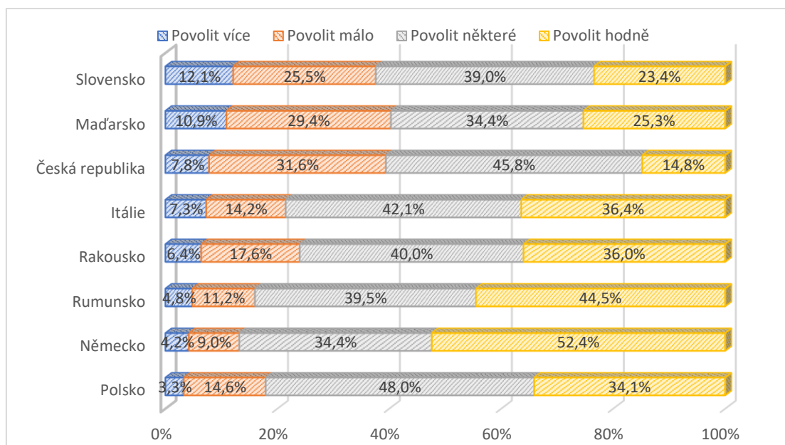
Graf 1 Postoj k přijímání ukrajinských uprchlíků
