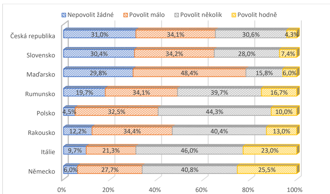
Graf 2 Postoj k přijímání syrských uprchlíků
