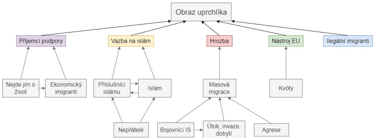
Schéma 1 Obraz uprchlíka v analyzovaném období evropské uprchlické krize
