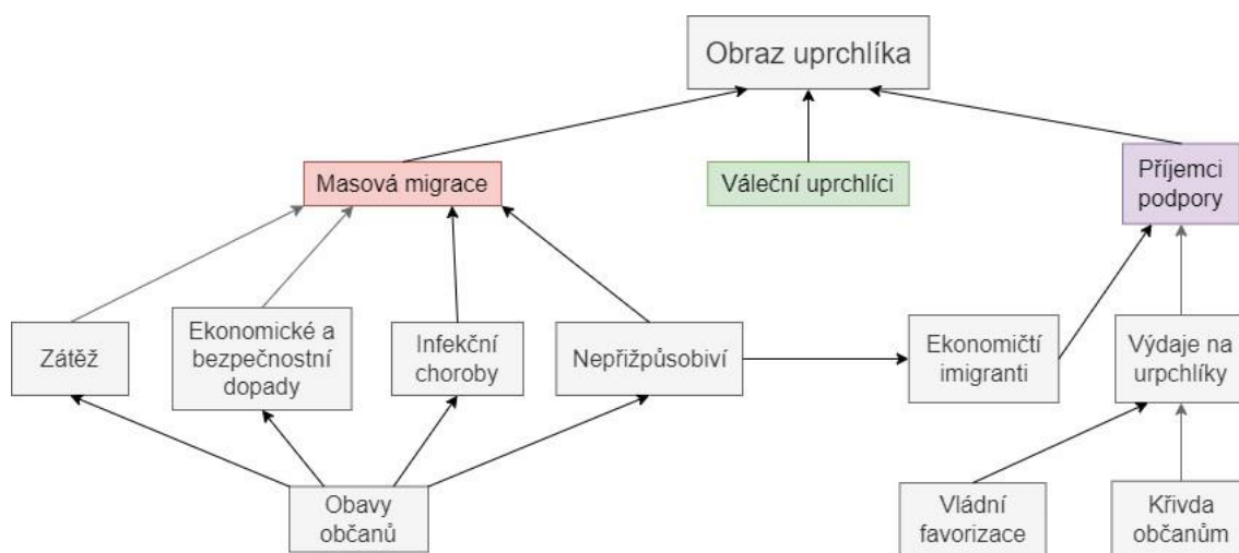
Schéma 2 Obraz uprchlíka v analyzovaném období ukrajinské uprchlické krize
