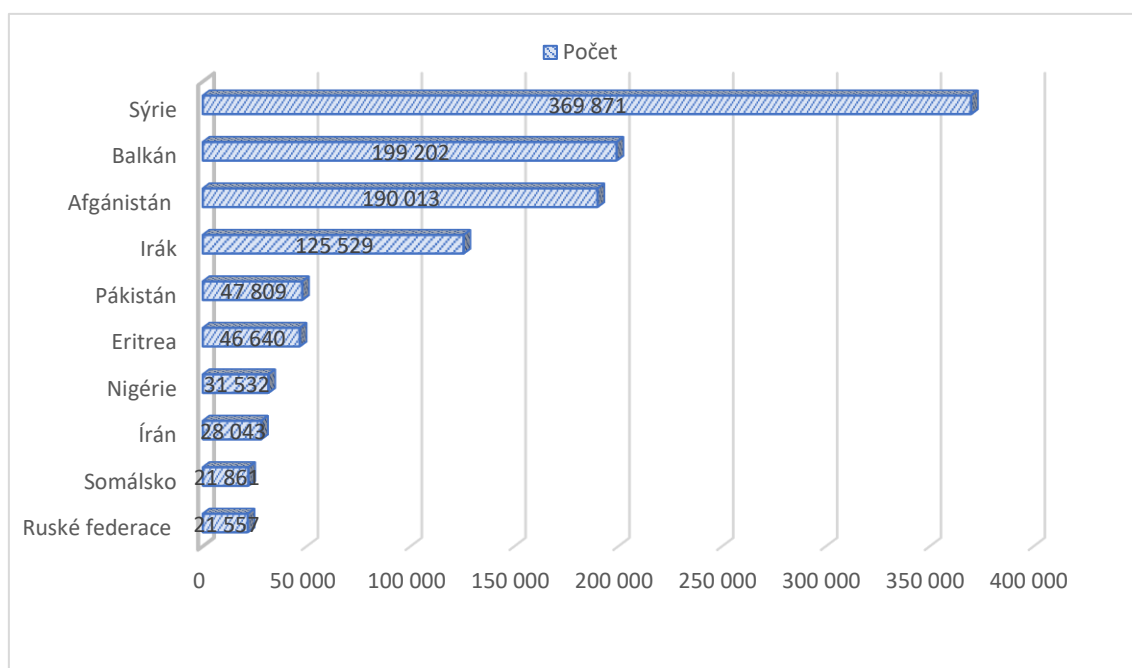
Graf 3 Hlavní země původu žadatelů o azyl v EU (2015)
