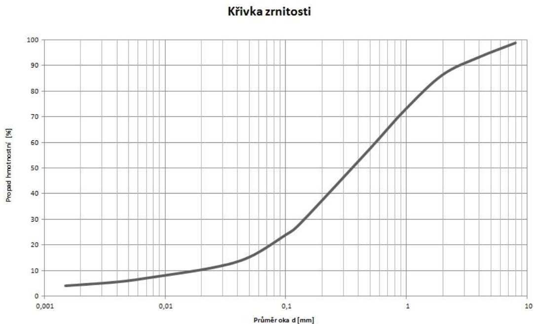
Obrázek 1 Křivka zrnitosti (převzato od Šobr, 2011)
