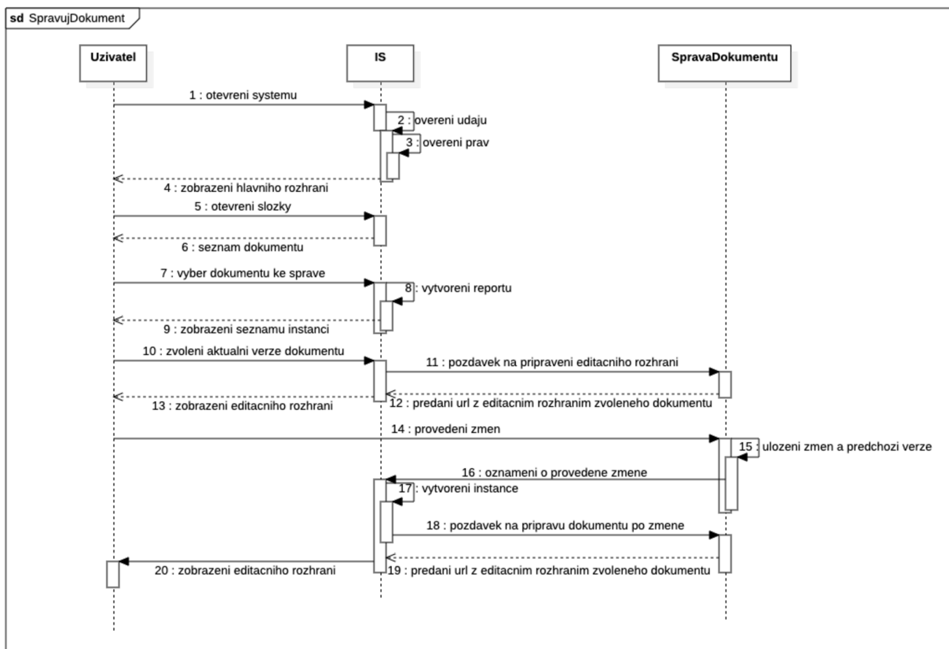
Obrázek 25 – Sekvenční diagram Spravuj dokument (Zdroj: Vlastní zpracování)
