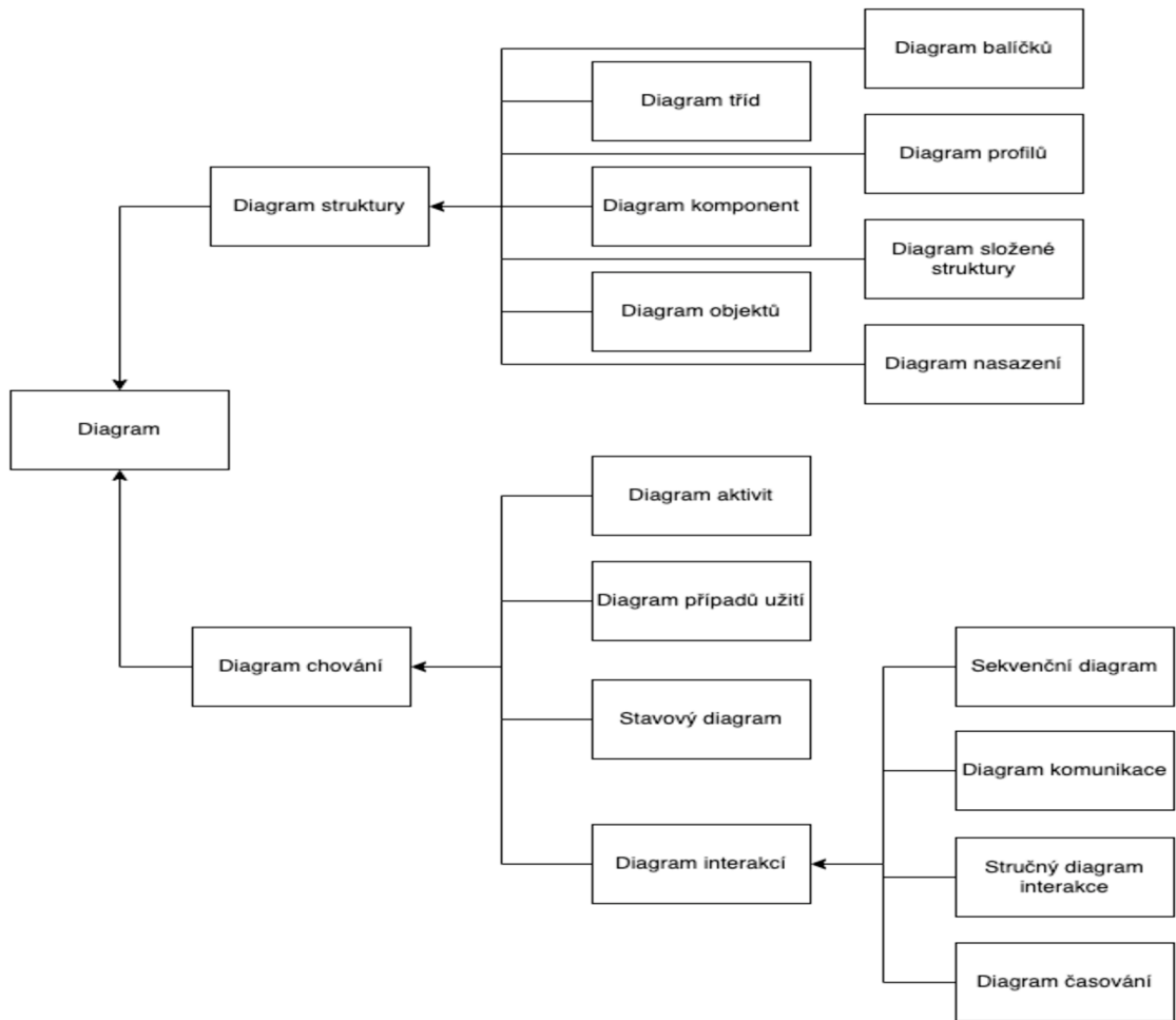
Obrázek 7 – Klasifikace diagramů UML (Zdroj: [28])
