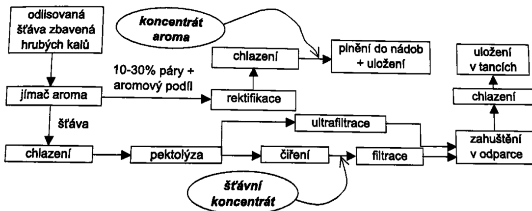
Obrázek 2: Schéma výroby šťávních koncentrátů (Kadlec et al. 2012)
