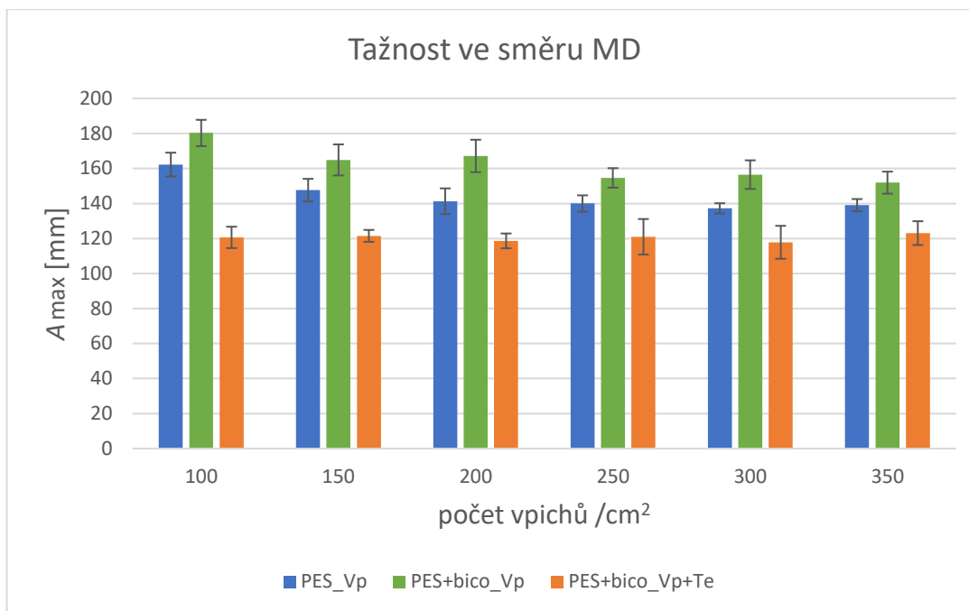
Obr. 39: Graf závislosti prodloužení ve směru MD.
