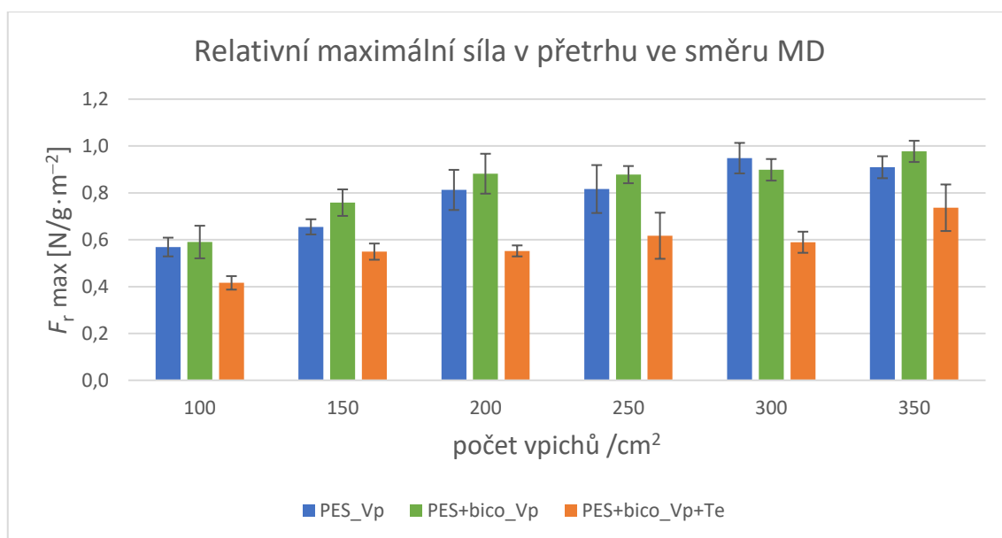
Obr. 37: Graf závislosti relativní maximální síly v přetrhu ve směru MD.
