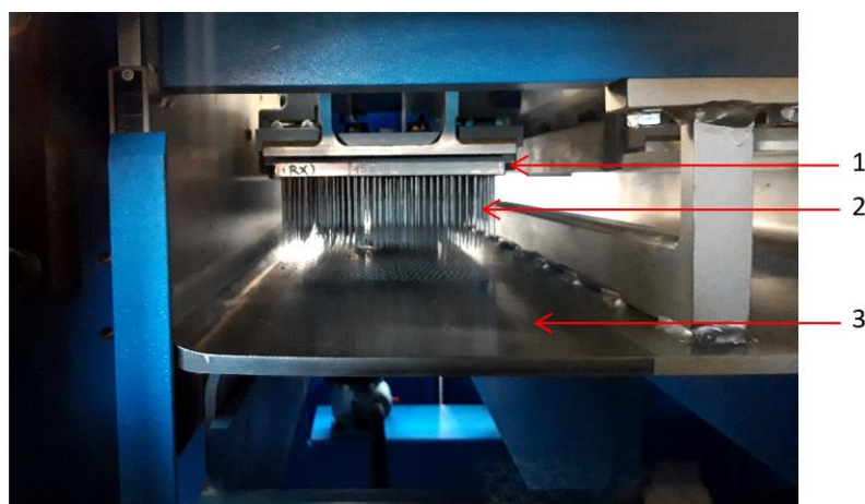
Obr. 26: Vpichovací stroj s jednou jehelní deskou. 1 – jehelní deska, 2 – vpichovací jehly, 3 – stírací rošt
