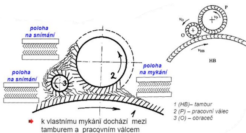
Obr. 5: Mykací uzel válcového stroje [16].
