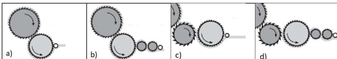
Obr. 6: Různé způsoby výroby vlákenné pavučiny mykáním [17].
