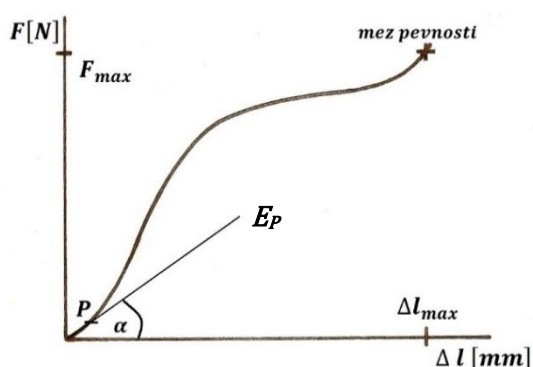
Obr. 21: Tahová křivka plošné textilie [22].
