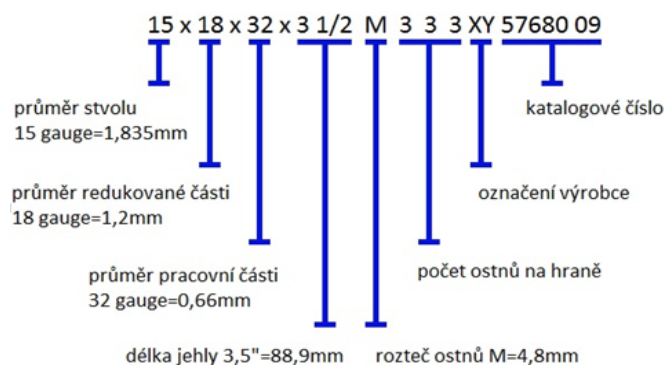
Obr. 16: Příklad značení jehly s redukovaným stvolem [15].
