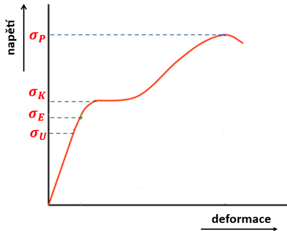
Obr. 20: Deformační křivka, závislost mezi napětím a deformací pevné látky [25].
