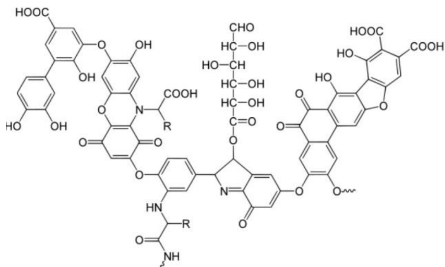
Obr. 1.1 Chemická struktura huminových kyselin
