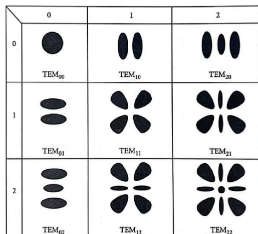
Obr 37 TEM módy paprsků [8]
