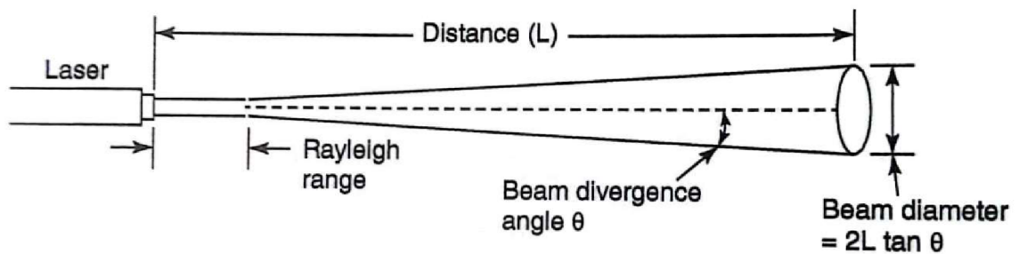
Obr 73 Znáornění rozbíhavosti (divergence) paprsku [2]
