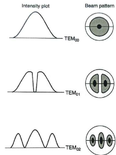
Obr 55 Znárodnění tvaru intenzity paprsku na Gaussově křivce [2]
