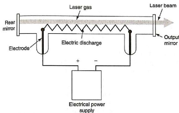
Obr 82 Buzení průchodem elektrického proudu [8]
