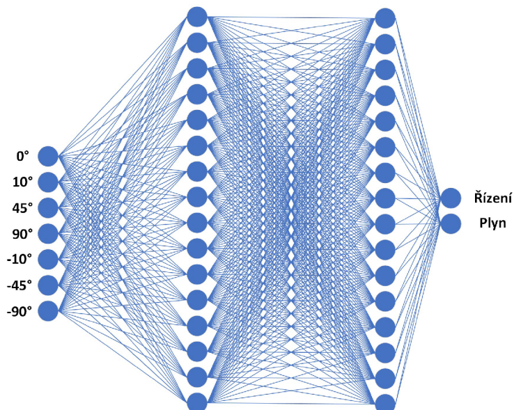
Obrázek 7: Neuronová síť 11
