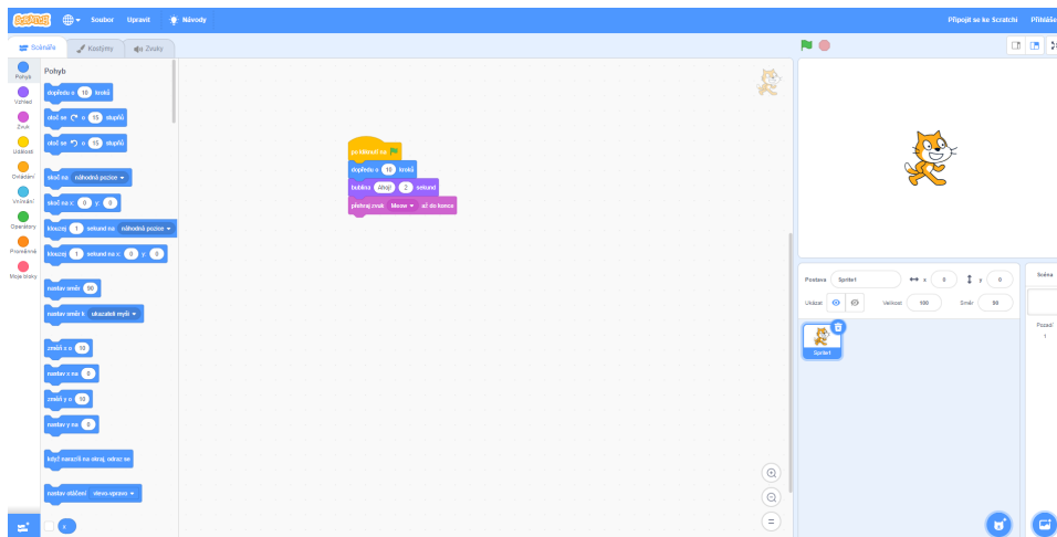
Obrázek 2.6: Prostředí Scratch
