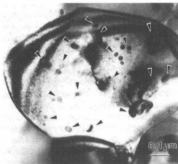
Obr. 3 TEM fotografie kompozitu Al 2 O 3 s 5 obj. % SiC (SiC je označen v obrázku černými šipkami). [13]
