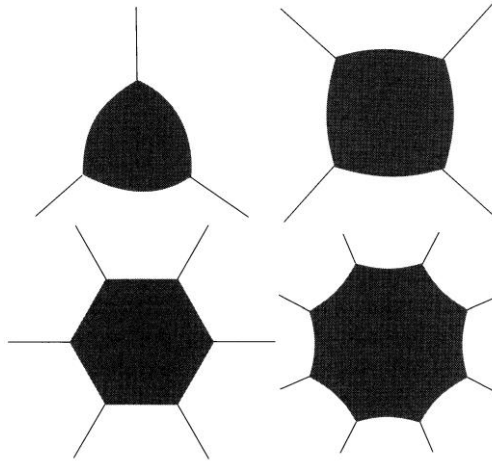
Obr. 12 Schéma zániku nebo růstu zrna (černá) podle počtu susedů (bílá). [1]
