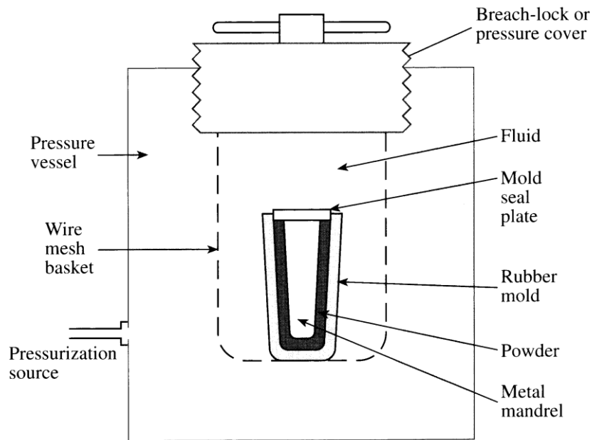
Obr. 8 Schéma izostatického lisování za studena (Breach-lock or pressure cover – přetlakový kryt, Fluid – tekutina, Mold seal plate – těsnicí destička formy, Rubber mold – gumová forma, Powder – prášek, Metal mandrel – kovový prášek, Pressure vessel – tlaková nádoba, Wire mesh basket – drátěný koš, Pressurization source – zdroj přetlaku). [1]
