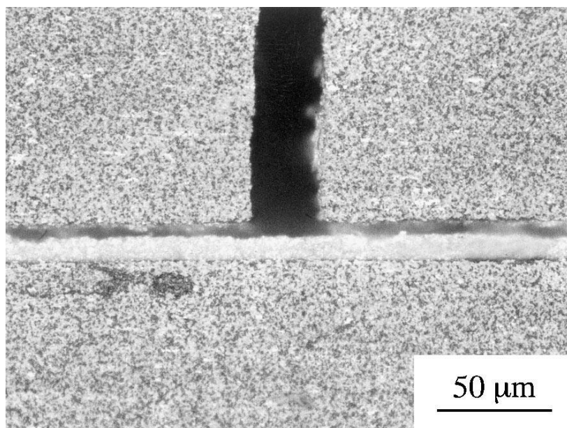
Obr. 5 SEM snímek šířící se trhliny skrz \text{Al}_2\text{O}_3 vrstvy a jejího odklonu do SiC vrstvy (delaminace laminátu). [18]
