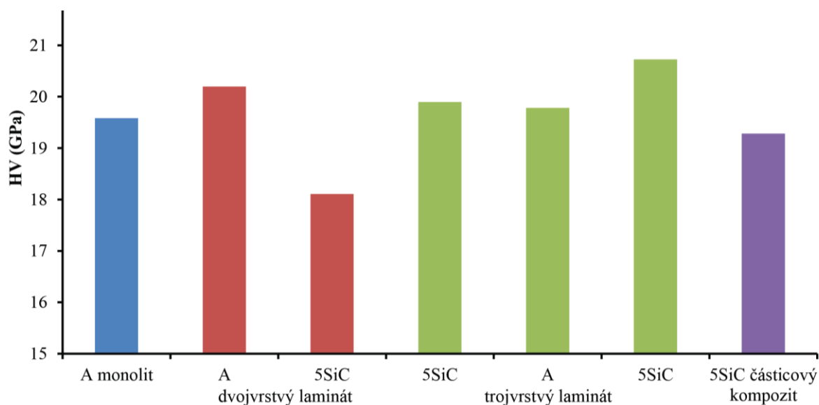
Obr. 24 Tvrdost slinutých disků čistého \text{Al}_2\text{O}_3 , 5SiC kompozitu a jednotlivých vrstev v laminátech.
