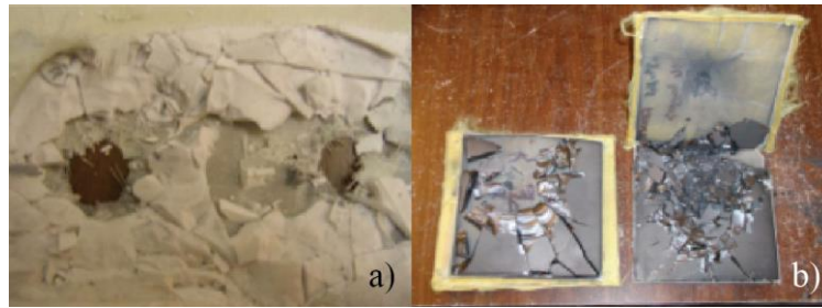
Obr. 16 Keramická destička po balistickém testování a) čisté \text{Al}_2\text{O}_3 , b) čisté \text{SiC} . [26]
