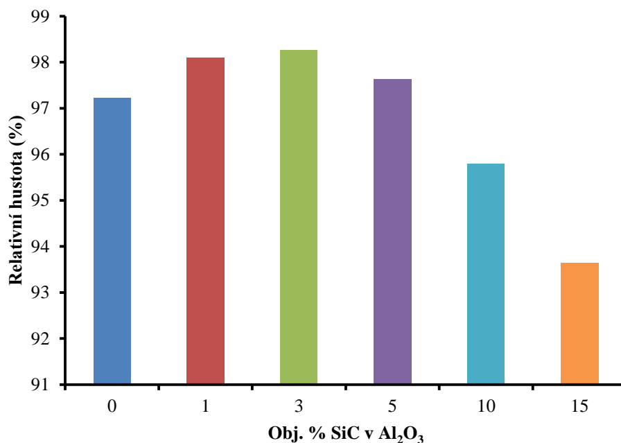
Obr. 18 Relativní hustota slinutých \text{Al}_2\text{O}_3 disků s různým přídavkem SiC ve struktuře připravených suchou cestou.
