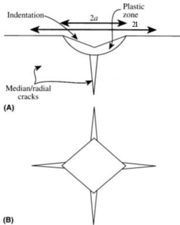
Obr. 15 Schéma indentačního vpichu s trhlinami. a) řez vpichem, b) půdorys vpichu. Indentation – vpich, Plastic zone – plastická zóna, Median/radial cracks – střední/radiální trhliny, 2a – délka úhlopříčky vpichu, 2l – délka radiálních trhlin vpichu. [1]
