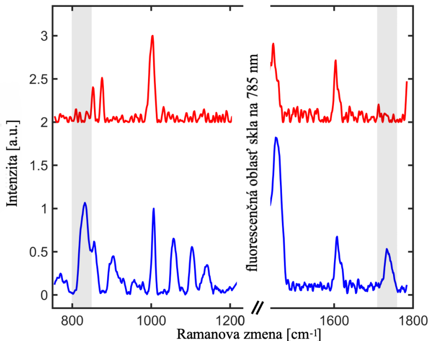
Obrázok 13: Dve Ramanovské spektrá zo zmesi, kde modrou farbou je opticky zachytený kmeň produkujúci PHB ( Cupriavidus necator H16) a červenou farbou je zachytená baktéria kmeňu neproduktujúceho PHB (spektrum bolo posunuté v smere osi y).
