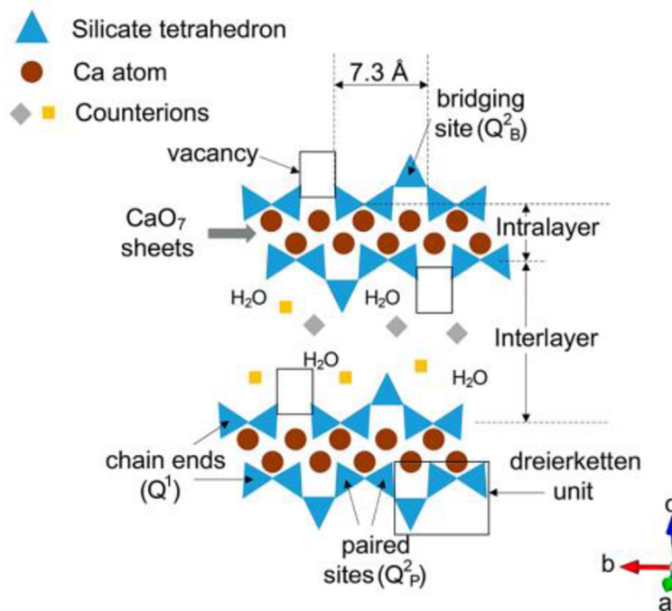
Obrázek 6 - Schematické znázornění nanostruktur C-S-H. Hnědé kruhy představují druhy Ca v Ca-O listu a modré trojúhelníky jsou silikátové jednotky v párových a přemosťujících místech. Šedá diamanty a žluté čtverce představují místa, která mohou být obsazena kationty, které náboj-neutralizují strukturu jako celek (např. Ca 2+ a/nebo K + ).[22]
