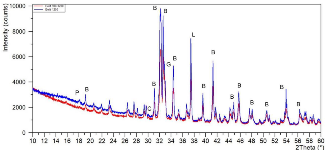
Obrázek č. 15. Difraktogram XRD analýzy – 900°C-1200°C x 1200°C s izoterm. výdrží 30 min
