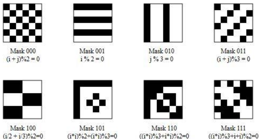
Obrázok 3.7 Maskovacie vzory pre QR kód [10]
