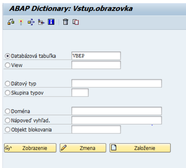
Obrázok 2.3 ABAP Dictionary
