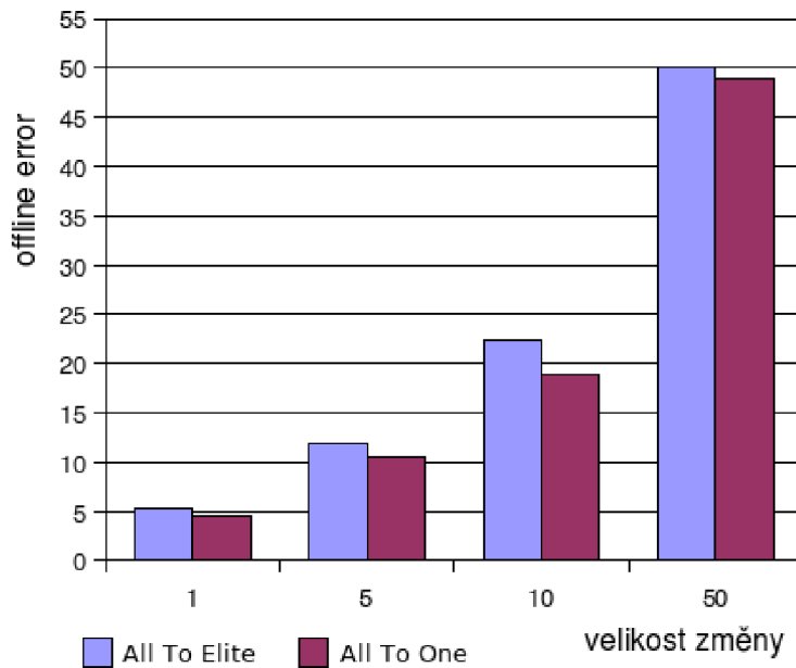
Obrázek 5.3: Graf offline error u strategií All To One a All To Elite pro různou velikost skoku vrcholů
