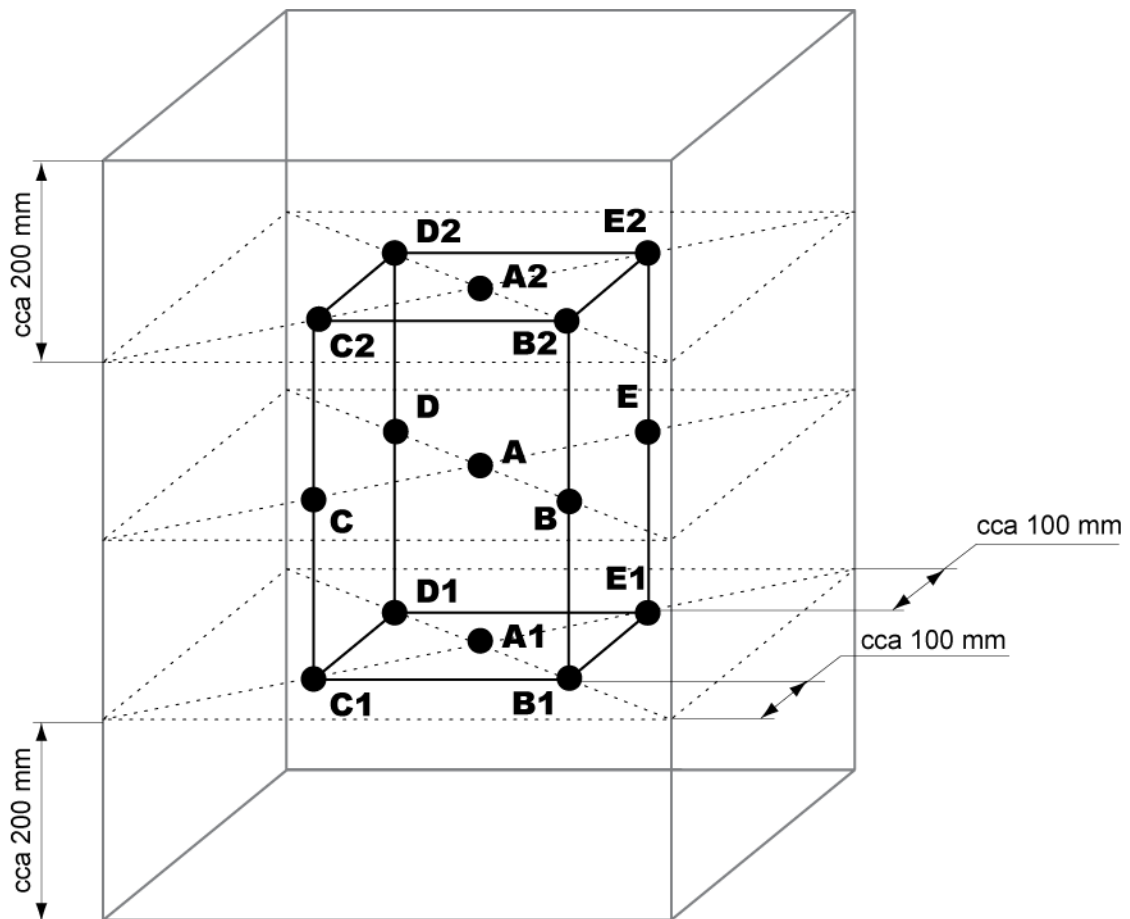
Obrázek 13 - Schéma měření
