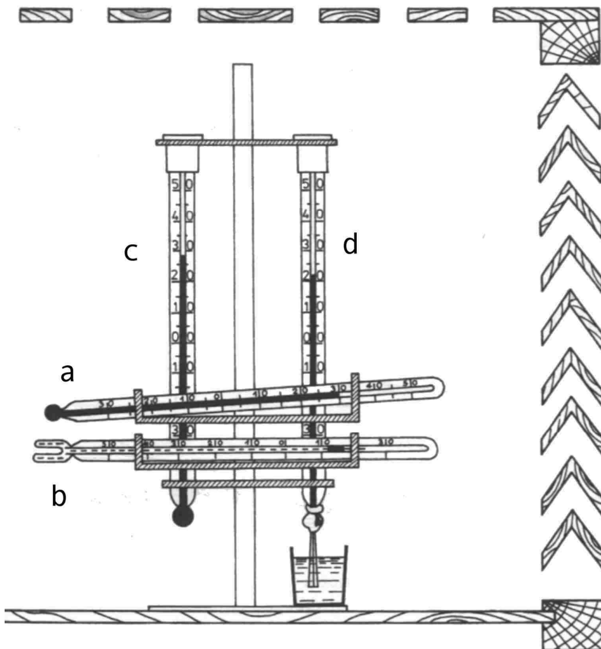
Obrázek 11 – Psychrometr
