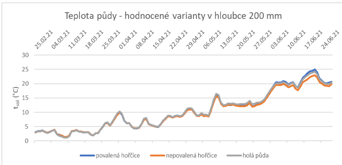
Graf 6: Průměrné hodnoty teploty půdy ( t_{soil} , °C) v hloubce půdy 200 mm na hodnocených variantách na lokalitě Kozojedy v období od 25. 2. 2021 až 28. 6. 2021.
