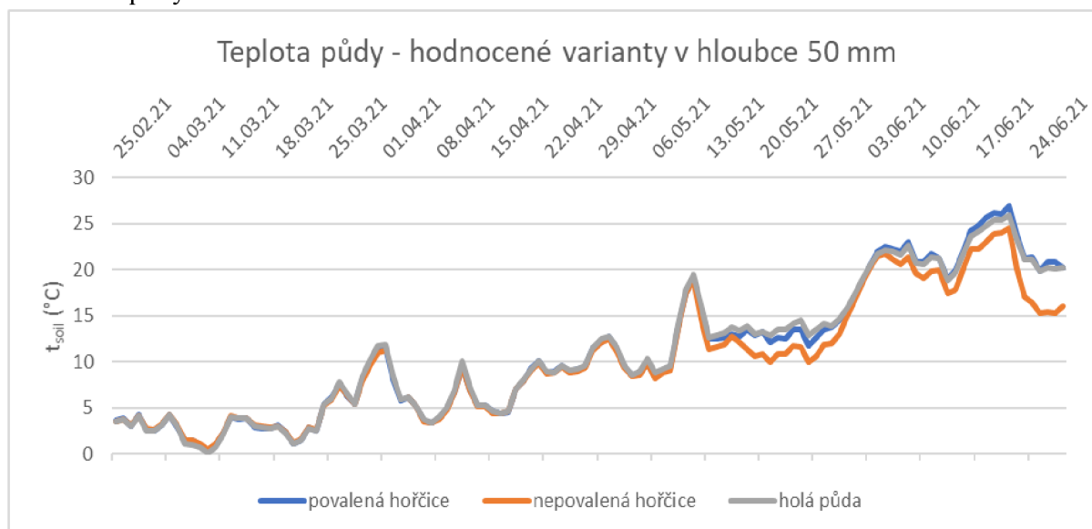
Graf 4: Průměrné hodnoty teploty půdy ( t_{soil} , °C) v hloubce půdy 50 mm na hodnocených variantách na lokalitě Kozojedy v období od 25. 2. 2021 až 28. 6. 2021.
