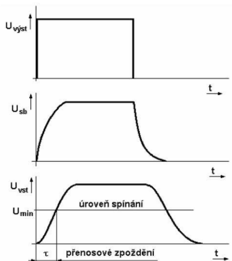
Obr. 17: Vznik přenosového signálu vlivem jeho deformace.[9]
