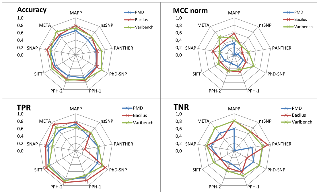
Obrázek 8.7: Komplexní srovnání nástrojů a nového META klasifikátoru.
