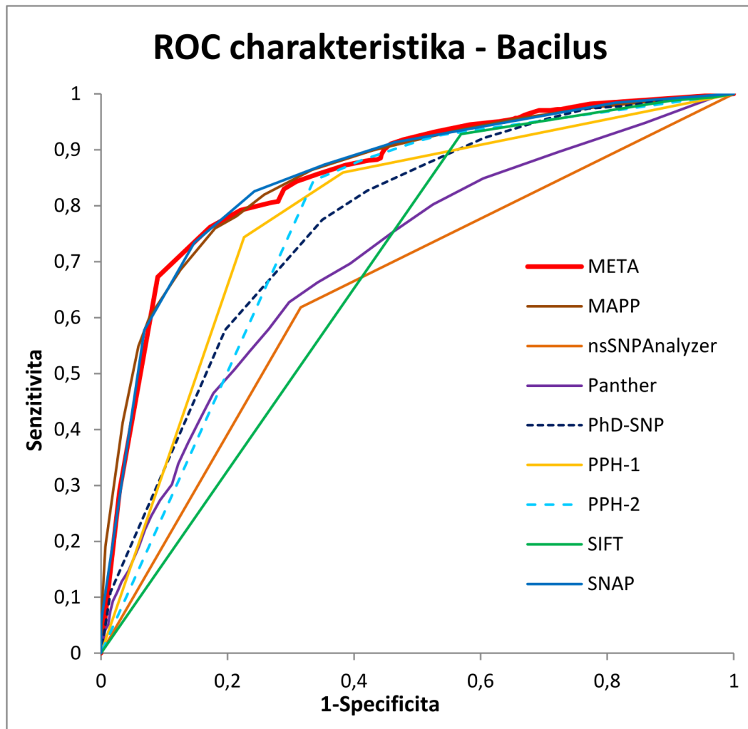
Obrázek 8.3: ROC charakteristiky nástrojů včetně nového klasifikátoru na sadě Bacilus.
