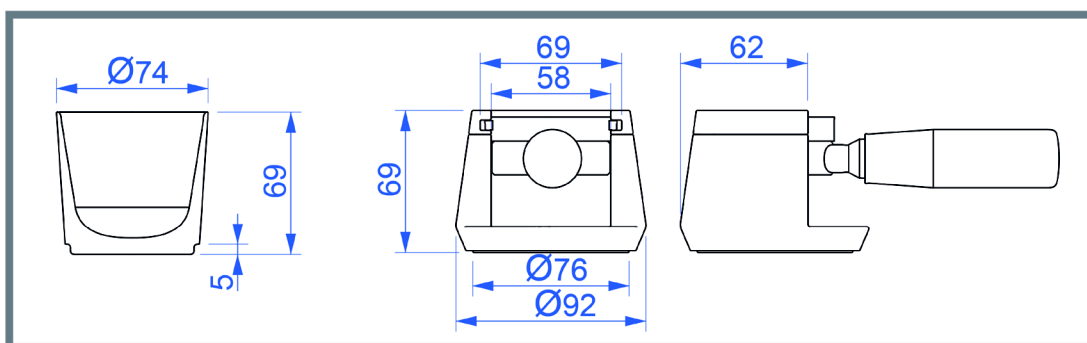
Obr. 5-6 Nákres kelímku a držáku
