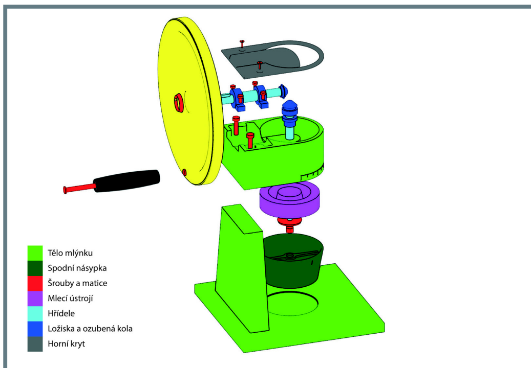
Obr. 5-2 Explodovaný pohled
