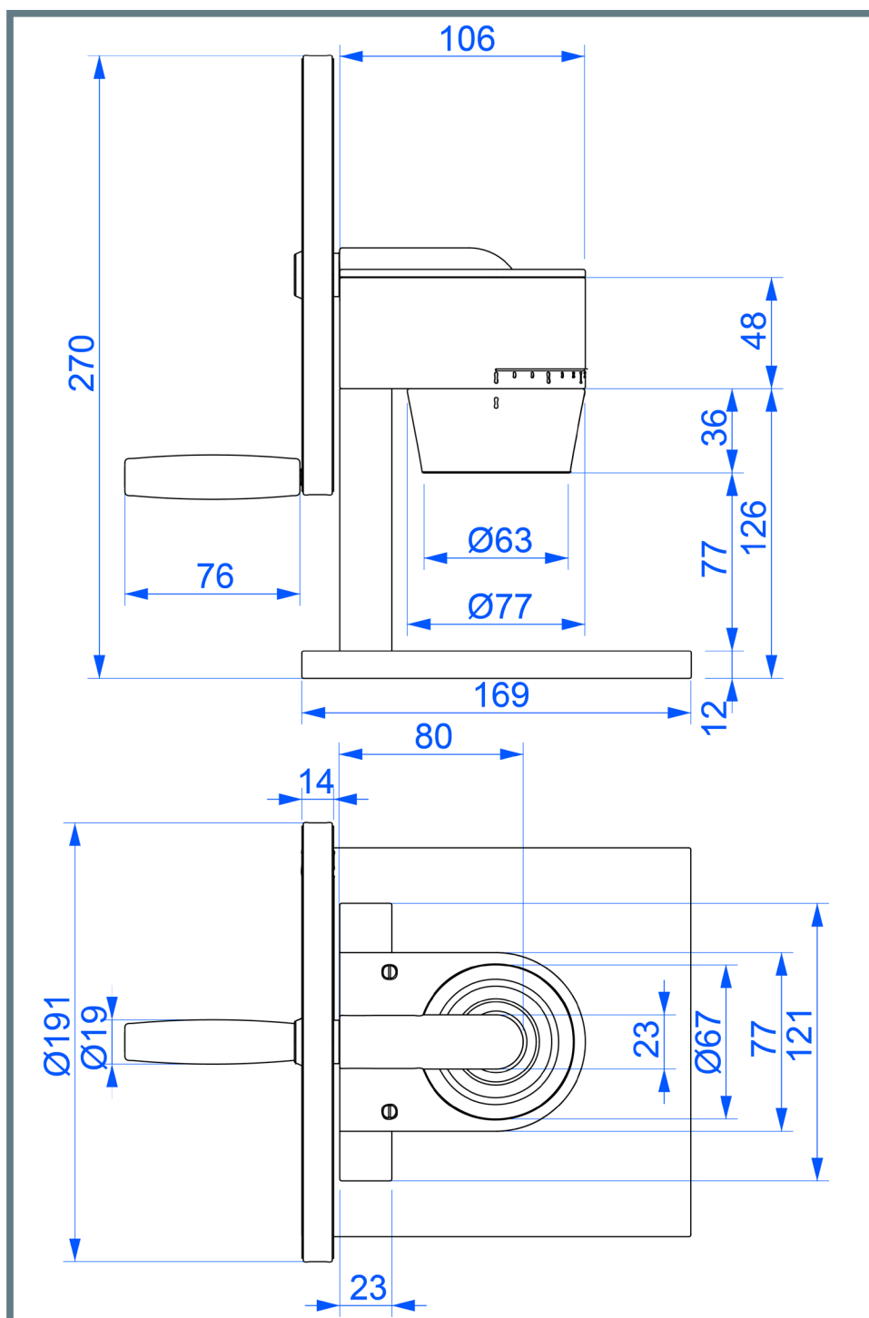
Obr.5-1 Rozměry mlýnku
