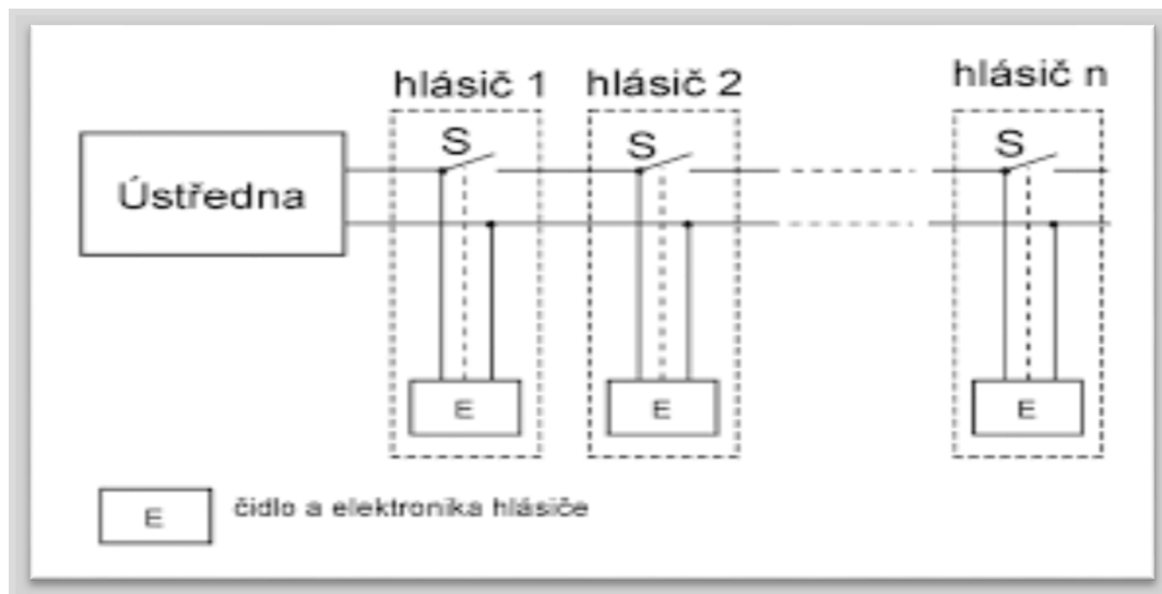
Obr. 11 – Blokové schéma-princip sériové adresace
