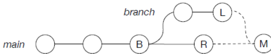
Obrázek 6: Sloučení větev v Git
