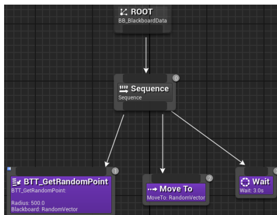
Obrázek 39: Dřevo chování pro patroly
