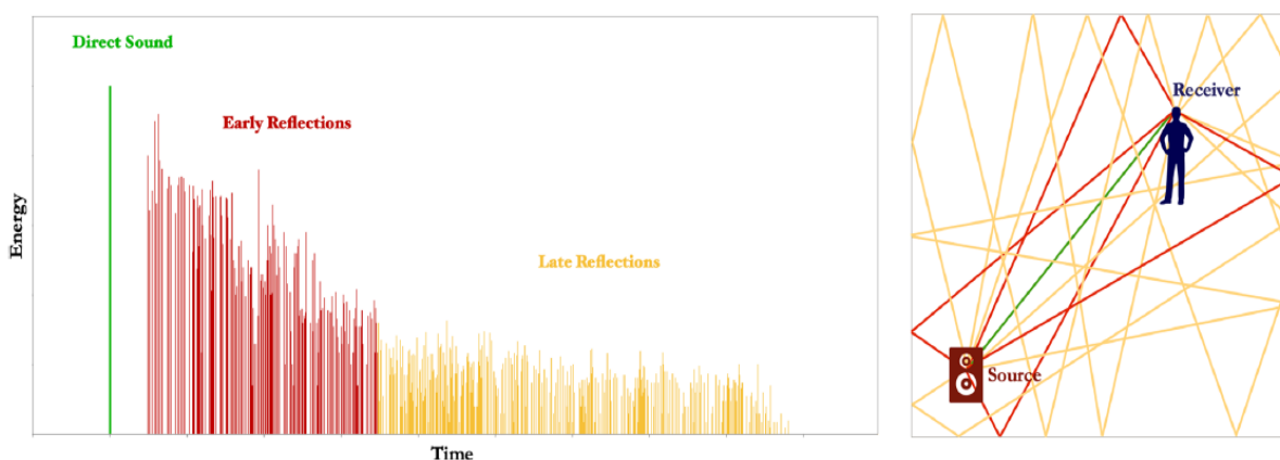
Obrázek 20: Přímý zvuk, ranní odrazy a pozdní reverberace
