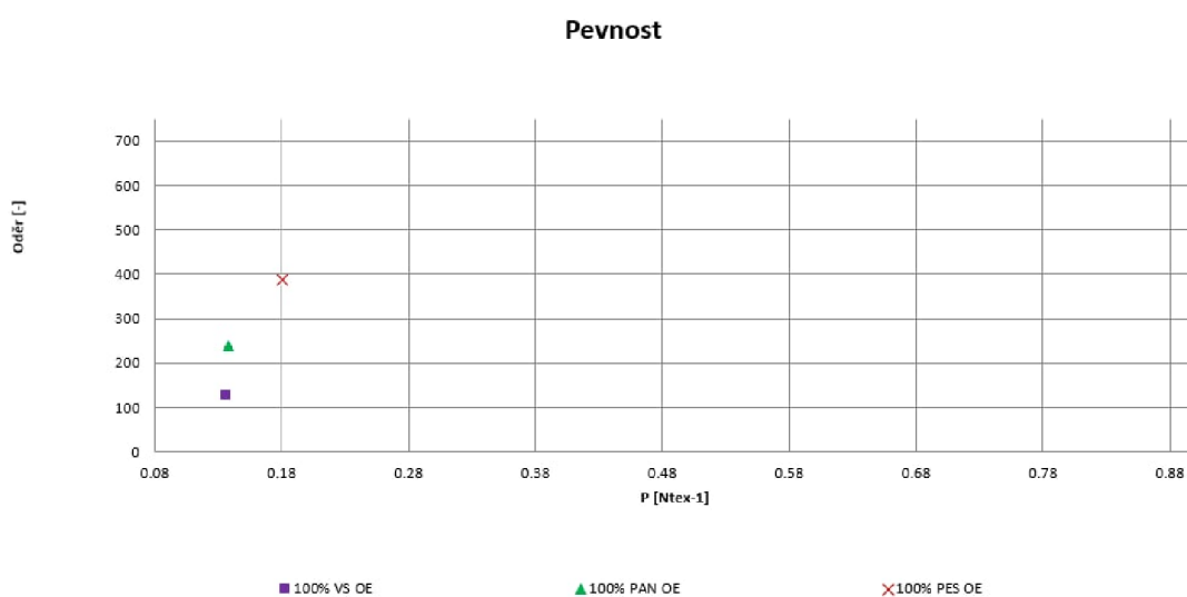
Obrázek graf č. 13 Vliv materiálu na pevnost.
