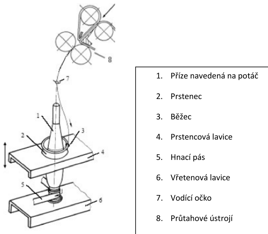
Obrázek č. 10 Schéma prstencového dopřádacího stroje [17]
