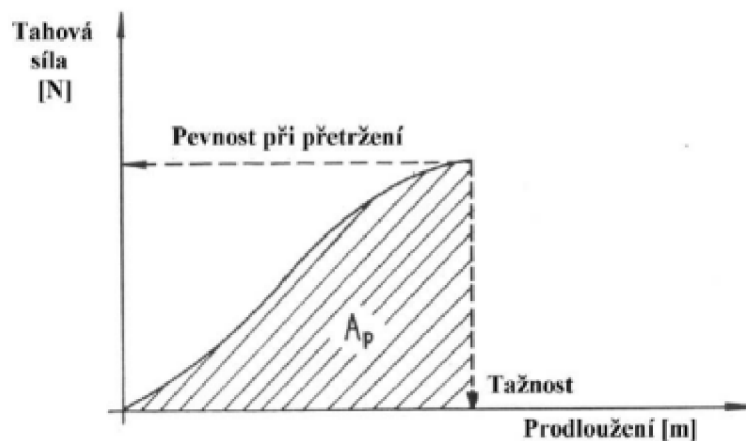
Obrázek č. 6 Graf znázornění závislosti pevnosti a tažnosti[9a]
