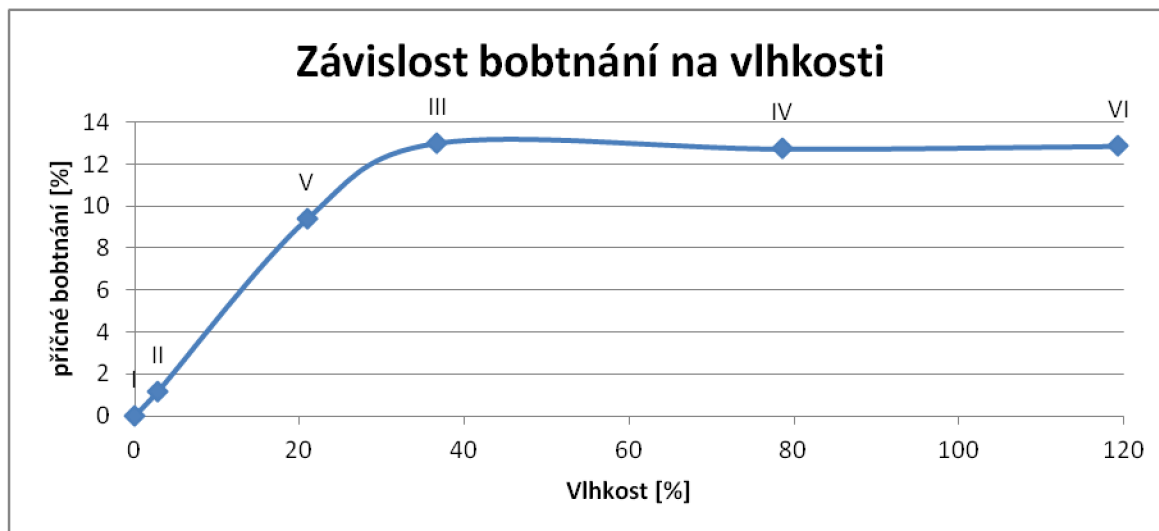
Graf 7: Závislost příčného bobtnání na vlhkosti
