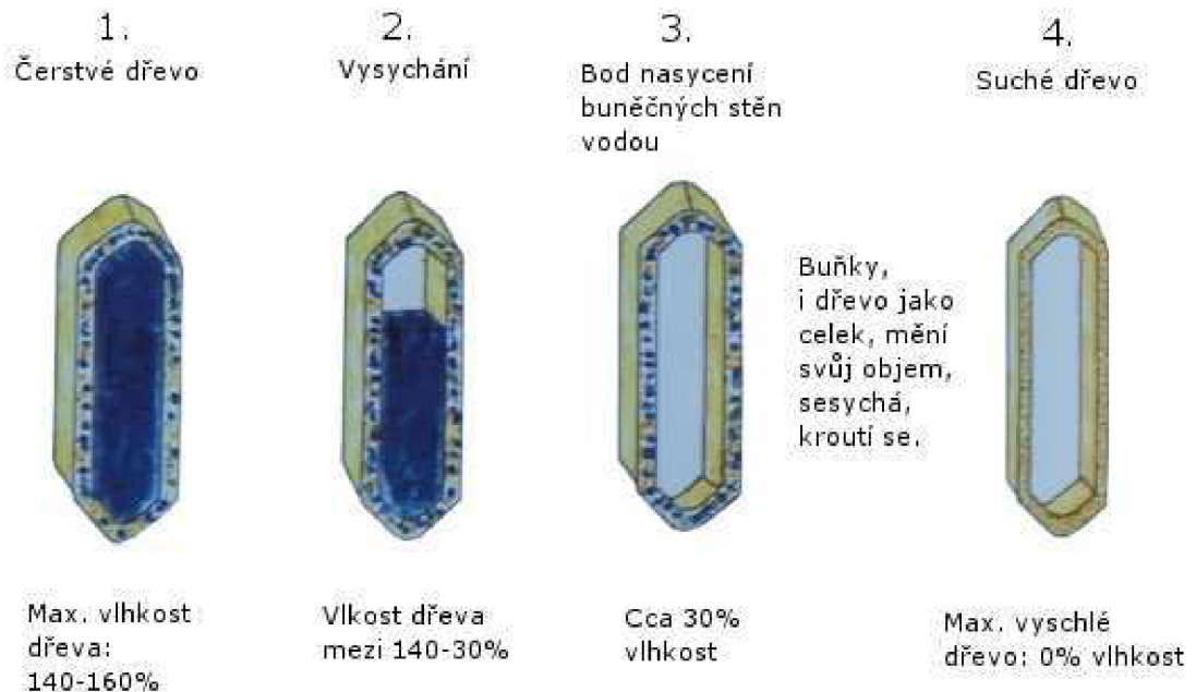
Obr. 5: Princip vysychání dřeva [15]
