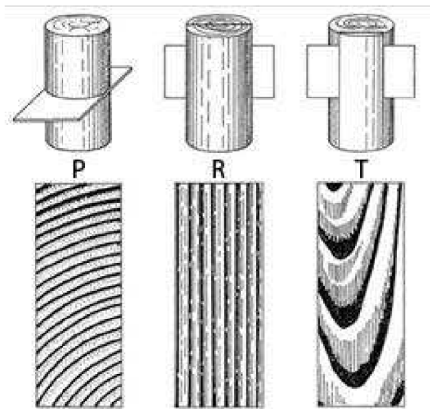
Obr. 2: Schéma základních řezů kmenem (příčný, radiální, tangenciální) [13]
